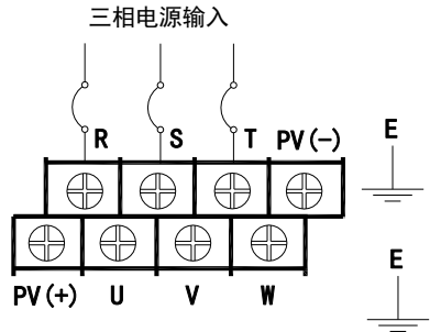
f) 75kW-110kW（T4/T5 电压等级）主回路端子排配线图
