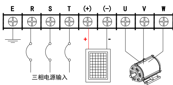
0.75kW-18.5kW（T4/T5 电压等级）主回路端子排配线图
