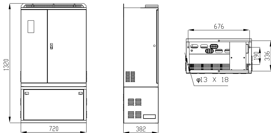
图 2-5 280kW~450kW (T4/T5 电压等级)落地安装示意图
