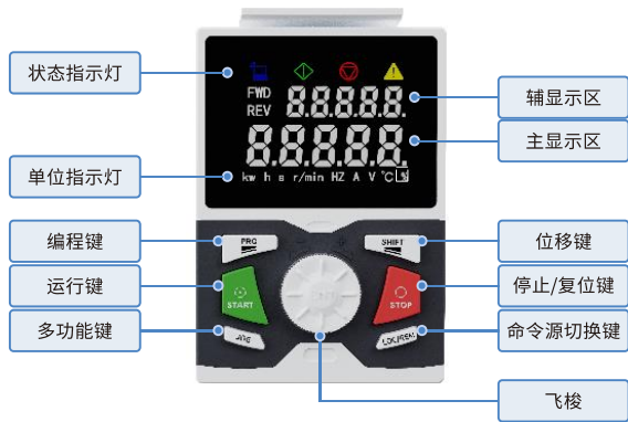
图 4-1 数码操作面板示意图
