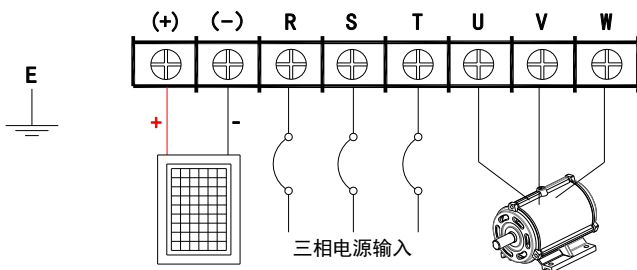
e) 55kW (T4/T5 电压等级) 主回路端子排配线图
