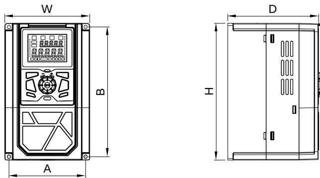
图 2-3 变频器壁挂安装示意图
