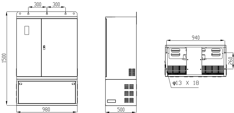
图 2-6 500kW~630kW (T4/T5 电压等级)落地安装示意图
