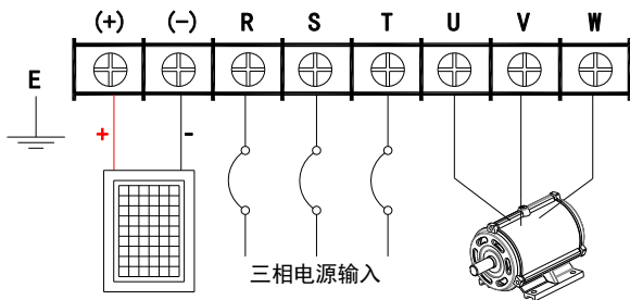
d) 37kW~45kW (T4/T5 电压等级) 主回路端子排配线图
