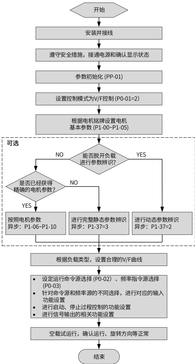
图 4-4 变频器调试流程图（V/F 控制）
