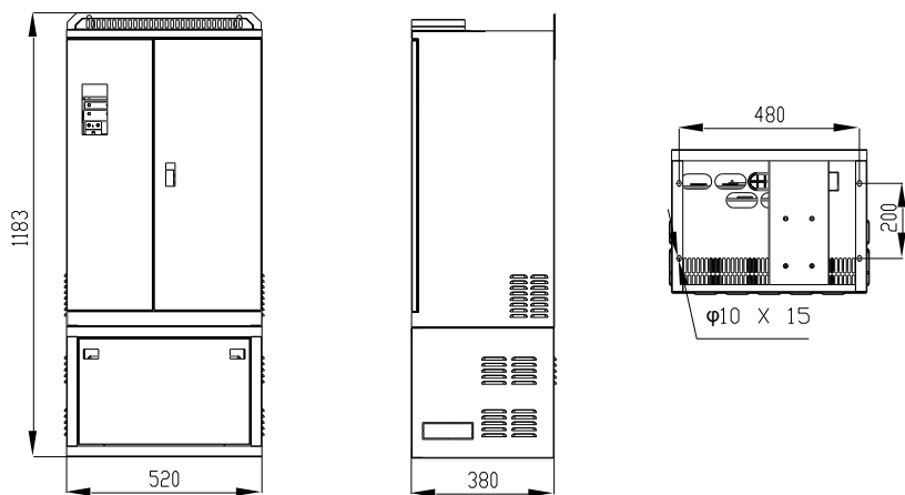
图 2-4 185kW~250kW (T4/T5 电压等级)落地安装示意图
