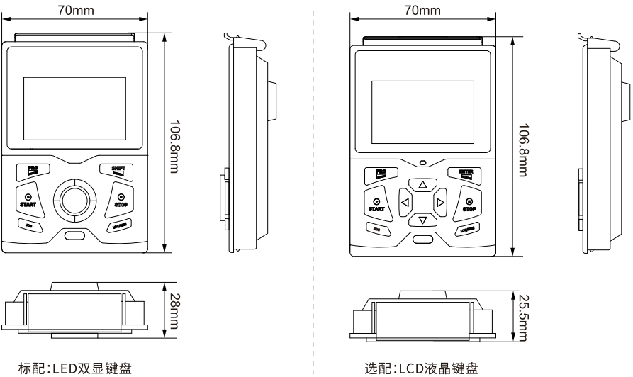
图 2-7 操作面板尺寸图
