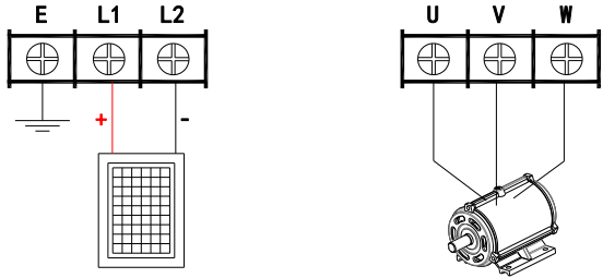
b) 3.7kW-7.5kW（T2 电压等级）主回路端子排配线图
