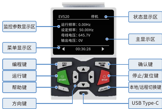
图 4-2 液晶操作面板示意图
