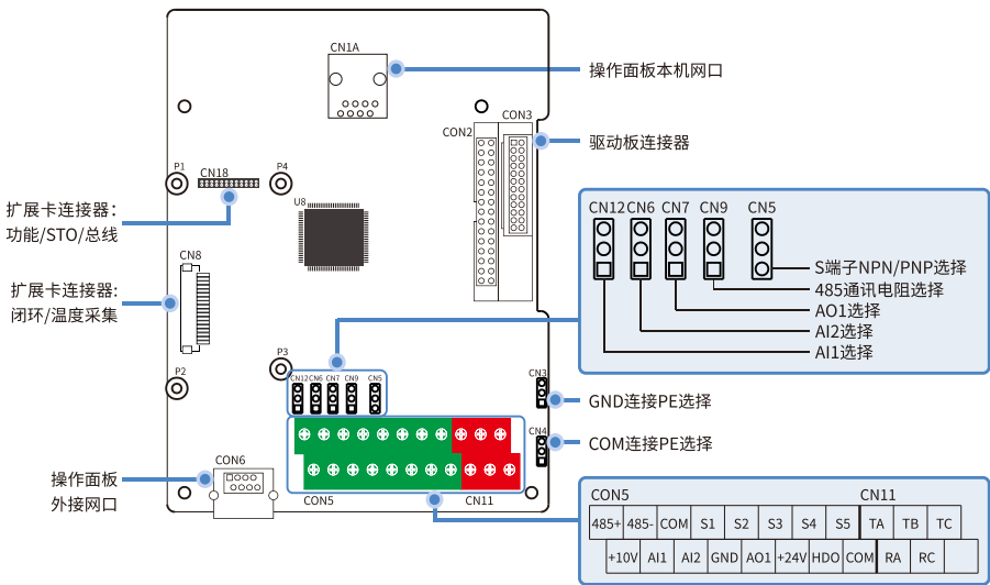
图 3-4 控制板端子分布图
