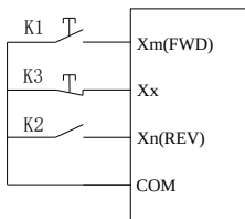
图 P4-5 三线式控制模式 2 示意图
