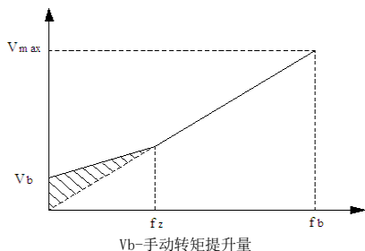
图 P3-1 转矩提升示意图
