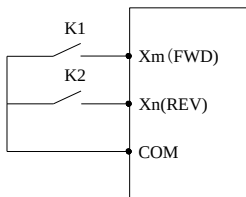
图 P4-2 二线式控制模式 1 示意图
