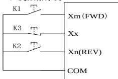
图 P4-4 三线式控制模式 1 示意图
