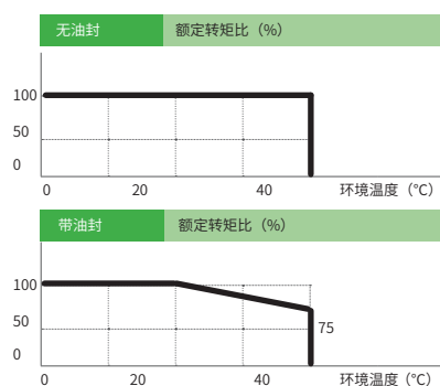
连续转矩 - 环境温度
