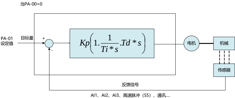
图 6-25 过程 PID 原理框图
