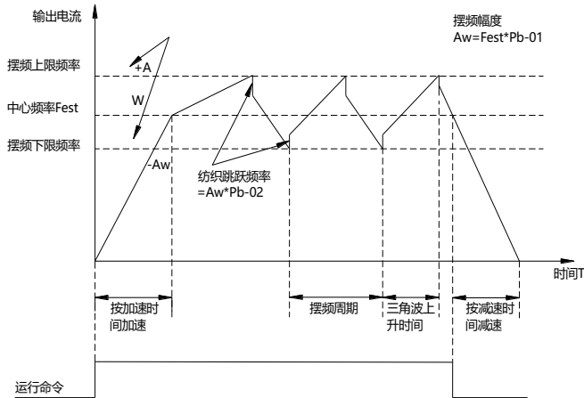
图 6-28 摆频工作示意图
