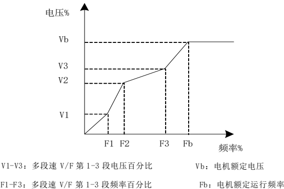
图 6-6 多点 V/F 曲线设定示意图
