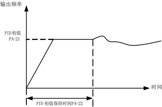
图 6-27 PID 初值的功能示意图
