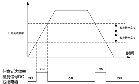
图 6-20 任意到达频率检测示意图
