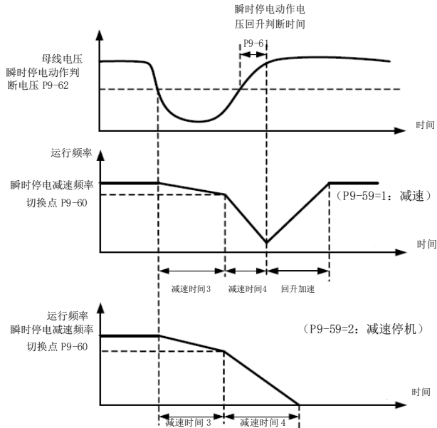
图 6-24 瞬时停电动作示意图
