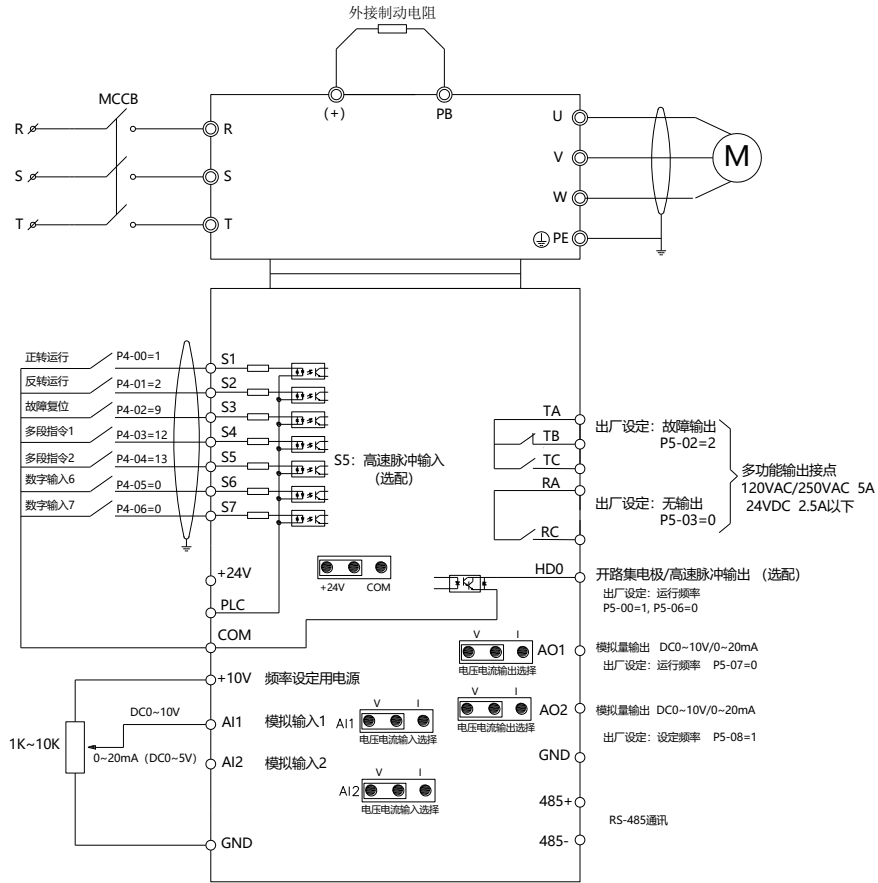
图 3-5 标准接线图
