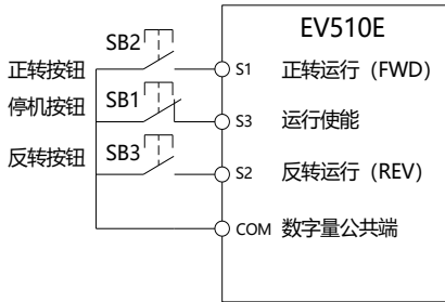
图 6-10 三线式控制模式 1
