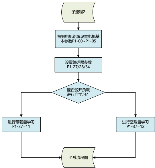
4. 2. 3. 驱动器调试子流程图 2
