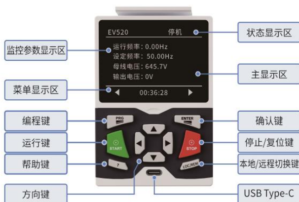
图 4-2 液晶操作面板示意图
