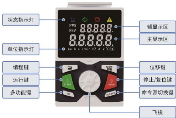
图 4-1 数码操作面板示意图
