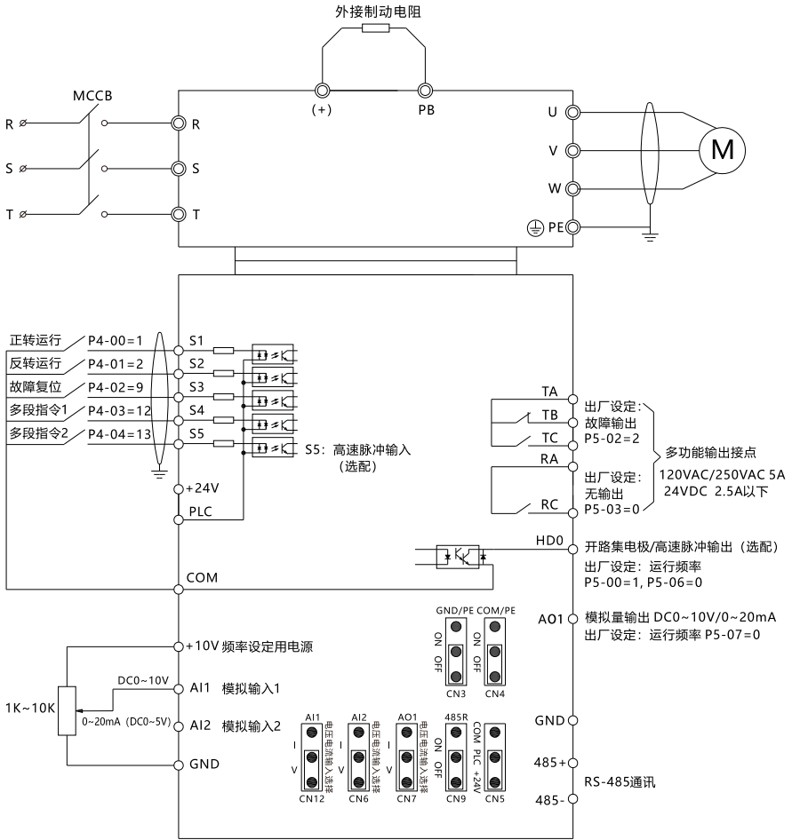
图 3-3 标准接线图
