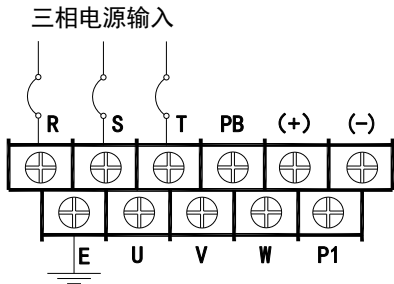
j) 500kW-630kW（T4/T5 电压等级）主回路端子排配线图
