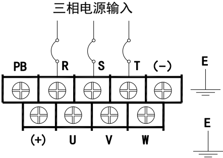
g) 132kW-160kW (T4/T5 电压等级) 主回路端子排配线图
