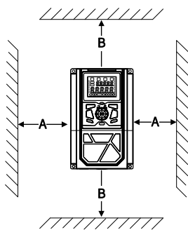
单体安装图
