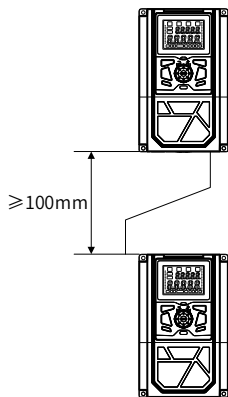
上下安装图
