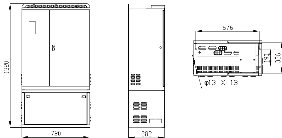
图 2-5 2800G/3150P~4500G (T4/T5 电压等级)落地安装示意图
