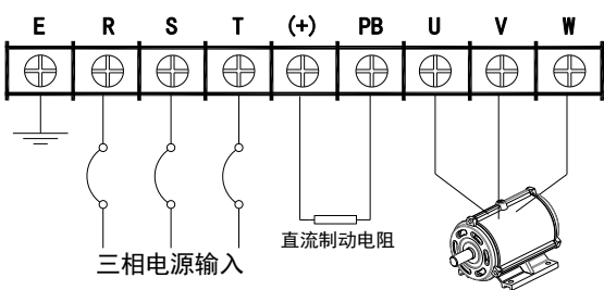
0.75kW-18.5kW (T4/T5 电压等级) 主回路端子排配线图
