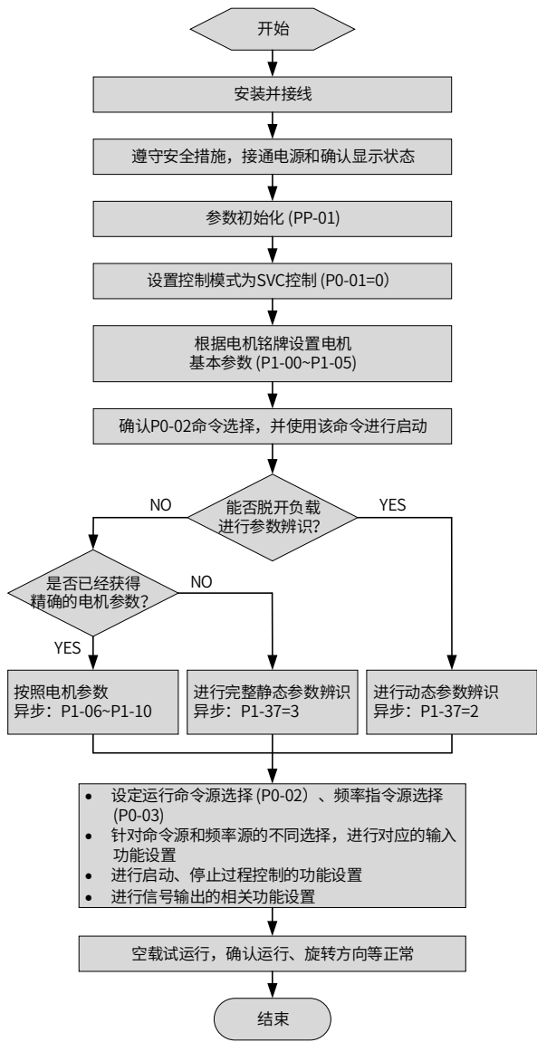
图 4-5 变频器调试流程图（SVC）
