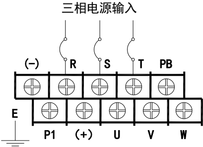
h) 185kW-250kW (T4/T5 电压等级) 主回路端子排配线图
