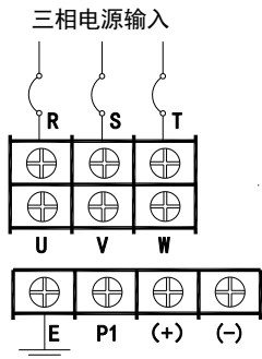
j) 500kW-630kW（T4/T5 电压等级）主回路端子排配线图
