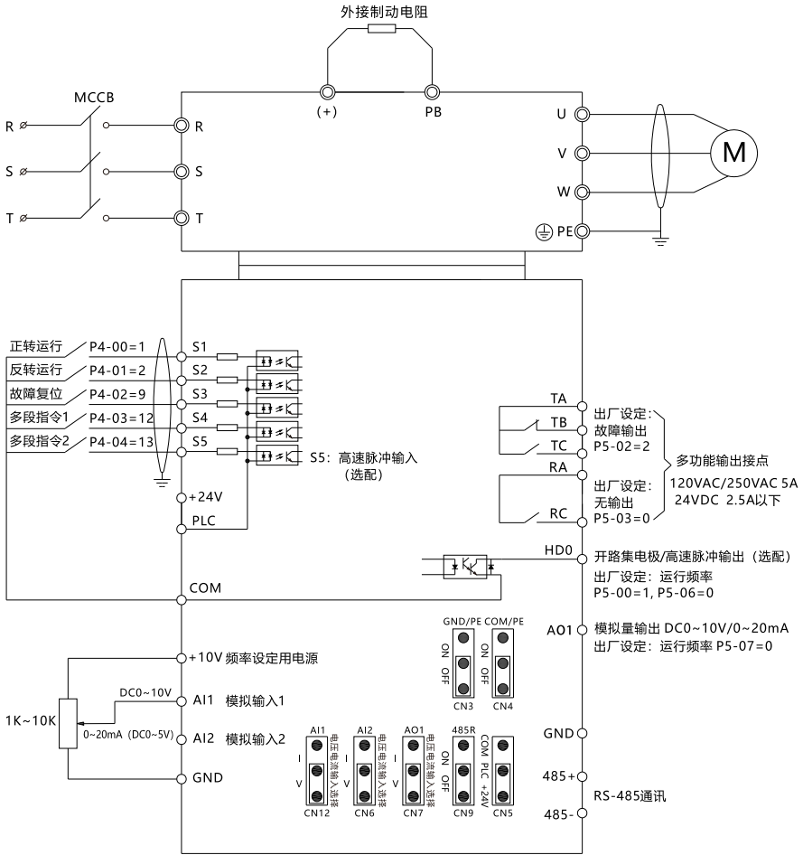
图 3-3 标准接线图
