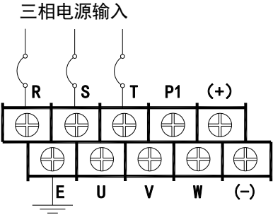
h) 185kW-250kW (T4/T5 电压等级) 主回路端子排配线图
