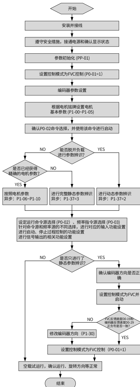
图 4-6 变频器调试流程图 (FVC)
