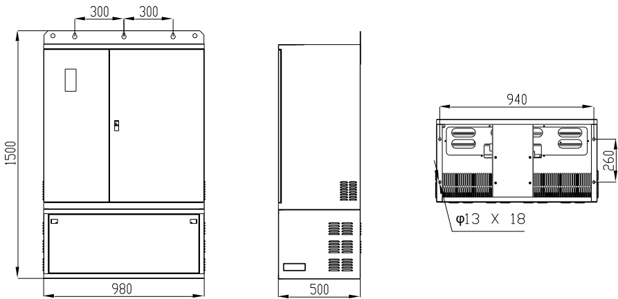
图 2-6 5000G~6300G (T4/T5 电压等级) 落地安装示意图
