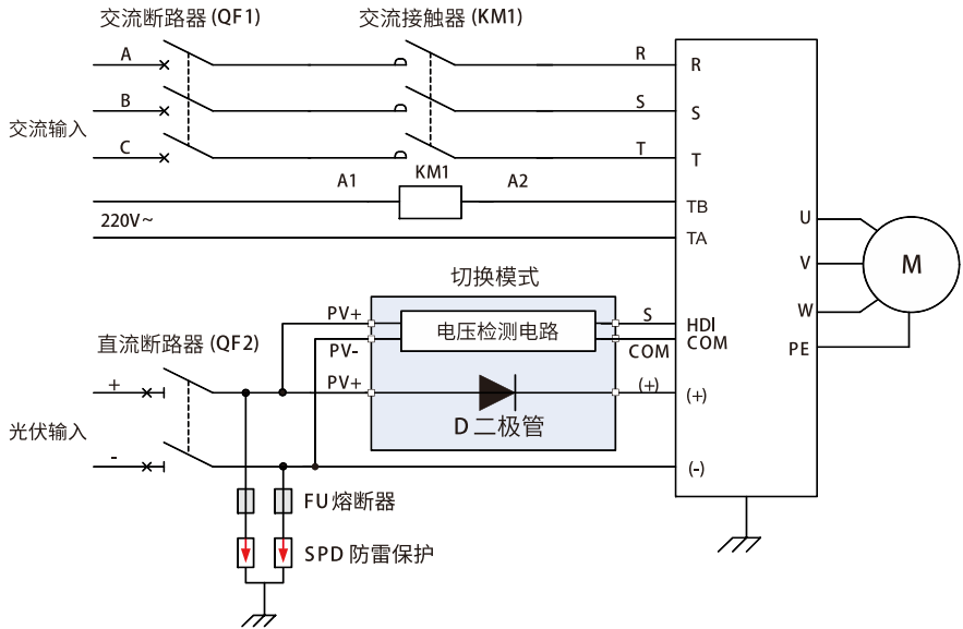
图 3-3 接线图
