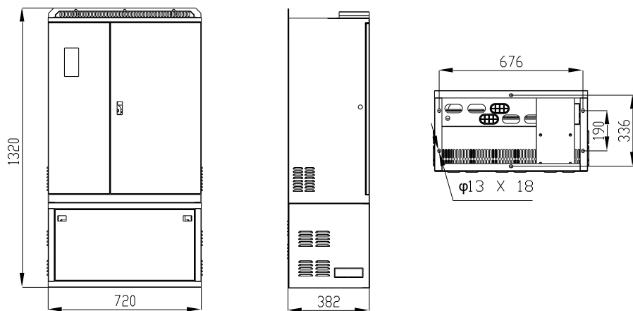
图 2-5 2800G~4500G (T4/T5 电压等级)落地安装示意图
