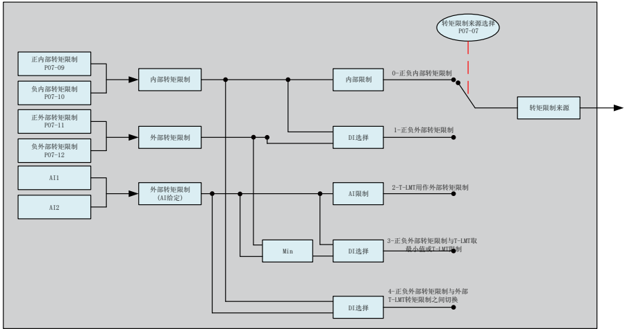
图 5-96 转矩限制来源
