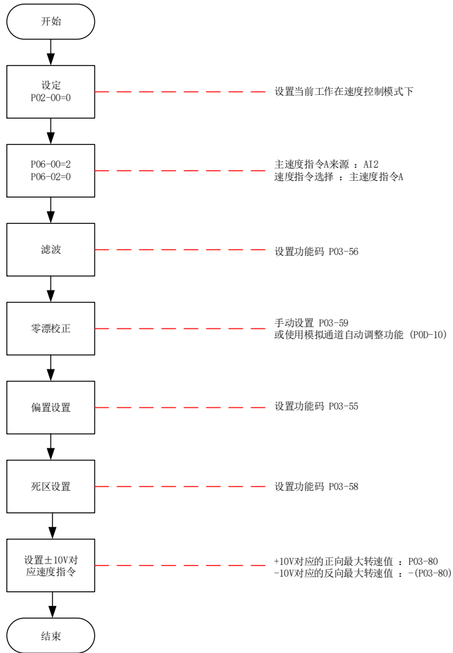
图 5-67 模拟量电压速度指令操作流程
