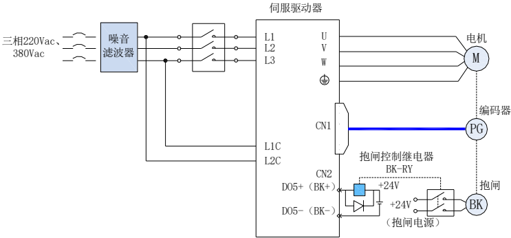
图 5-4 抱闸配线图
