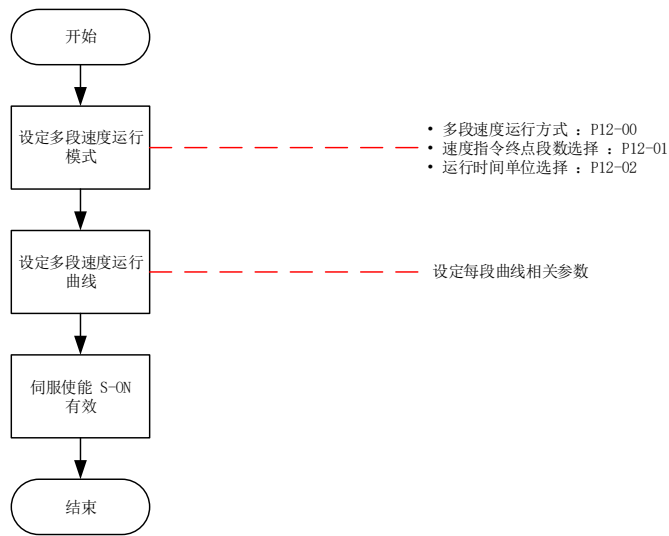
图 5-73 多段速度设置流程图
