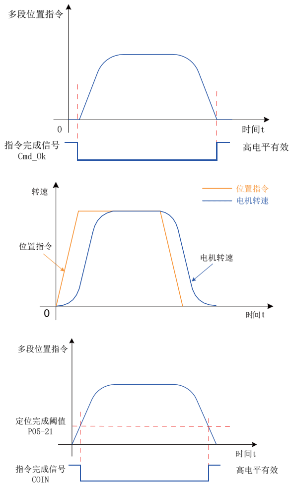
图 5-41 定位完成/接近功能说明
