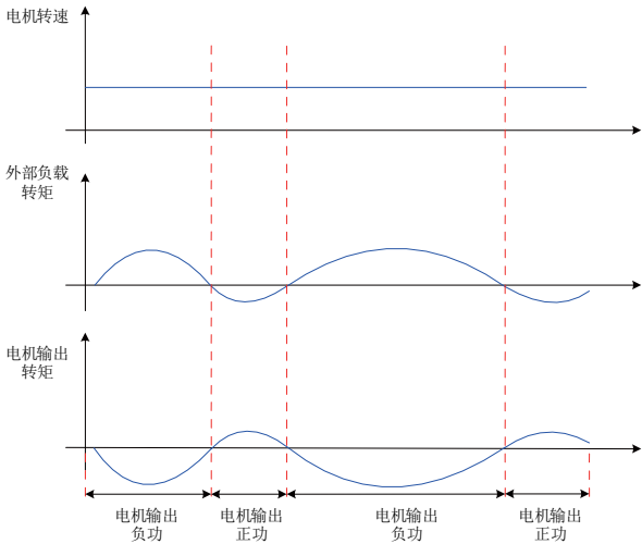
图 5-11 外部负载扭矩存在情况下曲线举例
