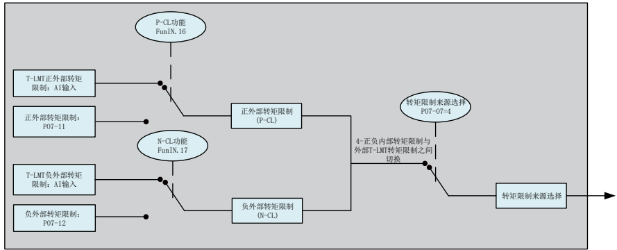
图 5-102 P07-07=4 转矩限制来源
