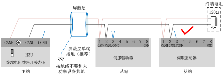
图 3-9 正确的 CAN 连接方法
