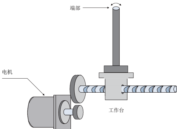
图 6-16 低频共振机械示意图
