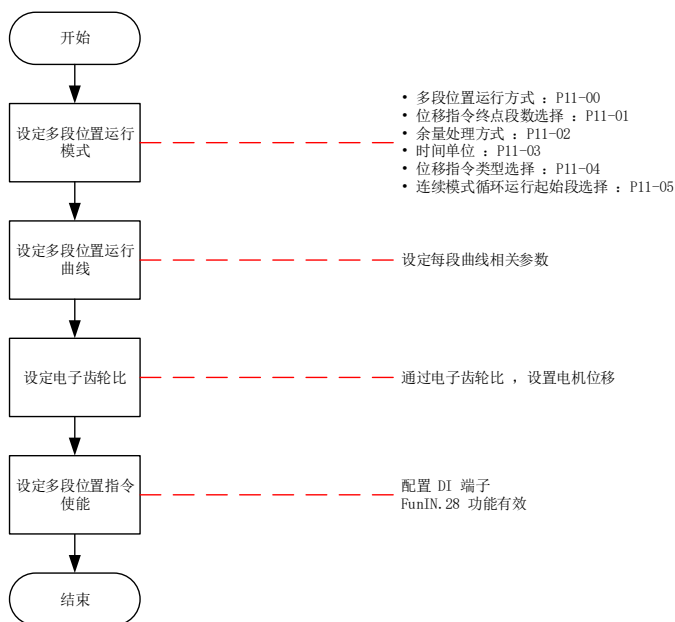
图 5-29 多段位置指令来源设置流程
