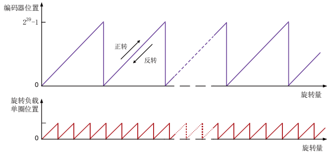
图 5-113 编码器反馈位置与旋转负载位置关系示意图
