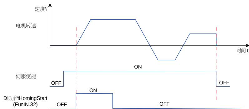
图 5-62 时序图举例
