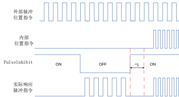
图 5-33 脉冲指令禁止功能波形举例
