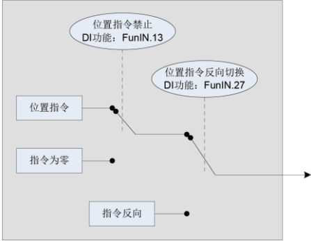
图 5-23 位置指令输入设置框图
