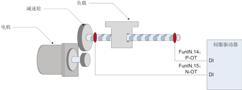
图 5-20 限位开关的安装示意图
