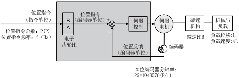
图 5-36 位置指令 (指令单位)、负载位移与电子齿轮比之间的关系
