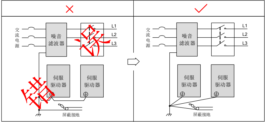
图 3-20 单点接地示意图
