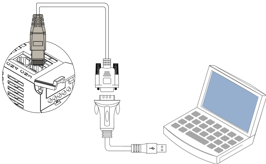
图 3-16 通信串口转 USB 示意图
