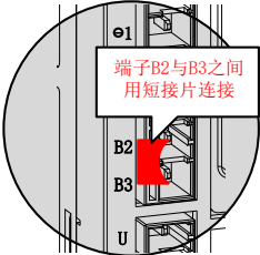
图 5-10 内置制动电阻使用短接片示意图
