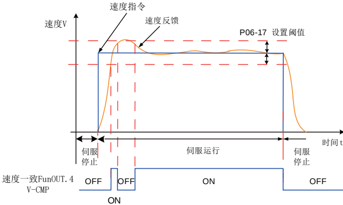
图 5-80 速度一致信号波形图
