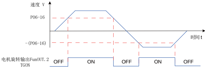
图 5-79 电机旋转信号波形图
