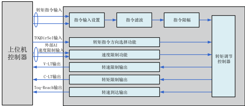
图 5-84 伺服驱动器与上位机信号交互图
