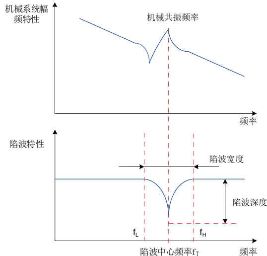
图 6-13 陷波器的抑制原理
