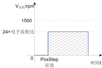
图 5-28 P05-00=1 时，电机运行曲线
