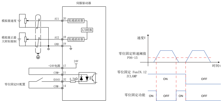
图 5-77 零位固定相关配线与波形图
