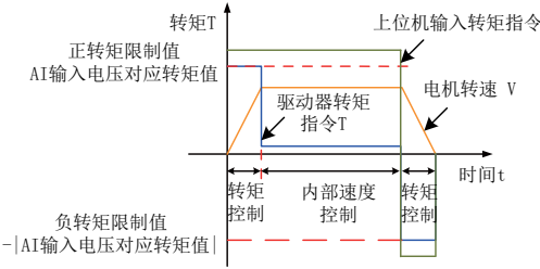
图 5-100 P07-07=2 转矩限制曲线图
