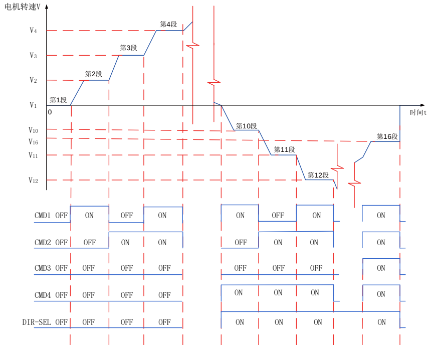
图 5-74 多段速度曲线举例
