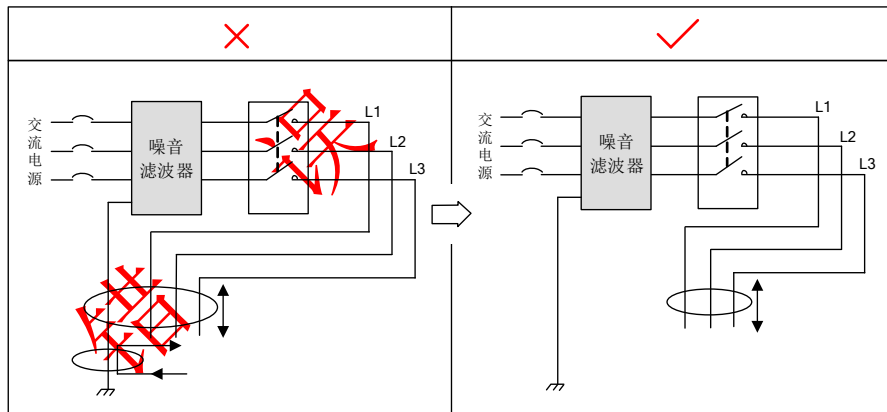
图 3-19 噪音滤波器地线与输出配线分离走线示意图
