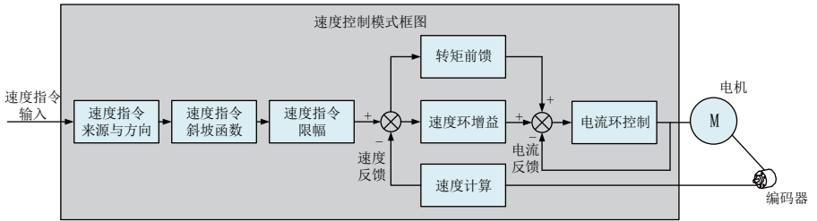
图 5-63 速度控制框图
