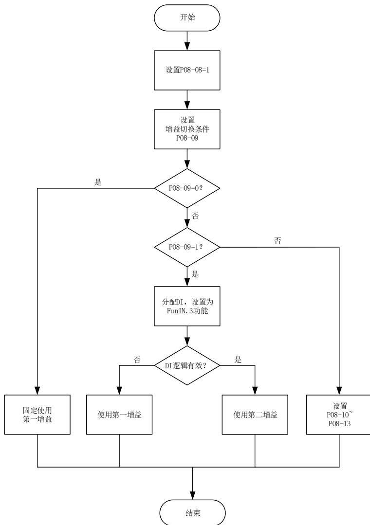
图 6-8 P08-08=1 增益切换流程图
