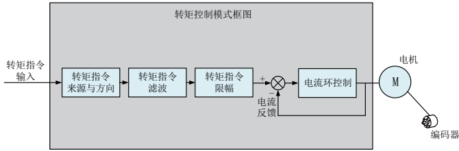
图 5-83 转矩控制框图
