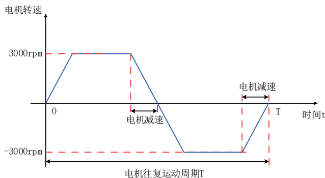
图 5-7 外部负载转矩不存在情况下电机速度曲线举例
