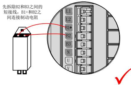
图 5-9 外接制动电阻连接示意图
