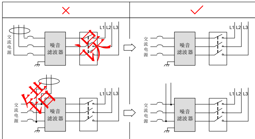
图 3-18 噪音滤波器输入与输出配线分离走线示意图
