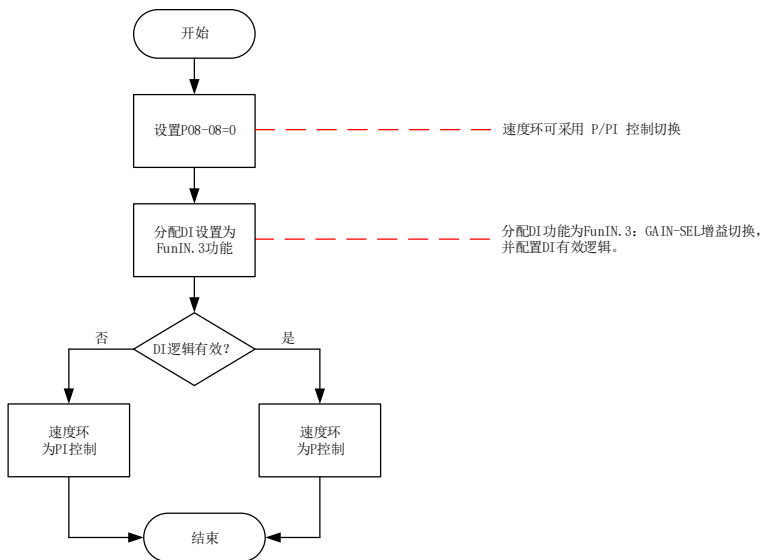
图 6-7 P08-08=0 增益切换流程图
