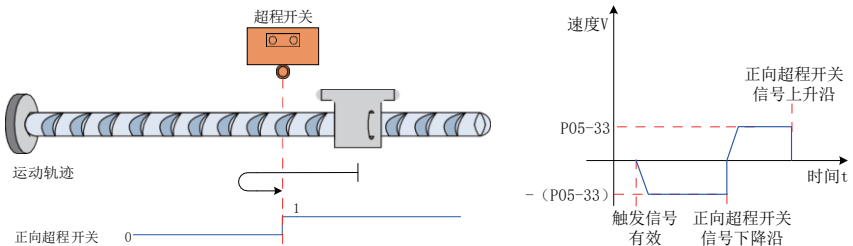
图 5-56 模式 6 原点回零电机运行曲线②与转速说明
