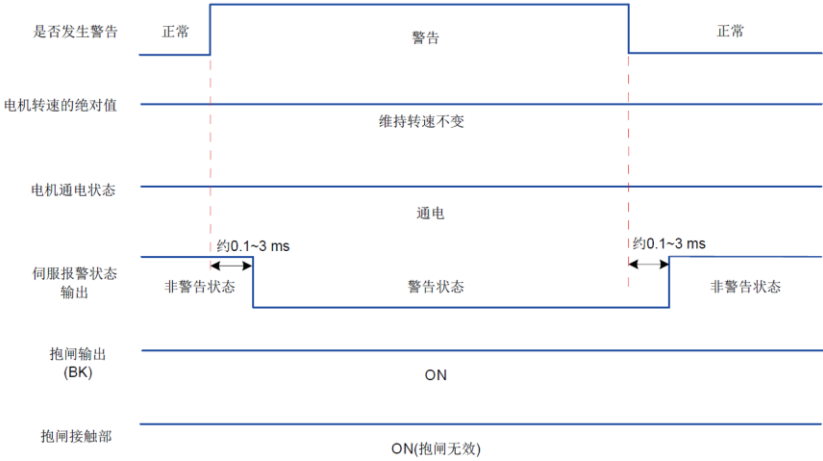
图 5-18 非停机警告时序图
