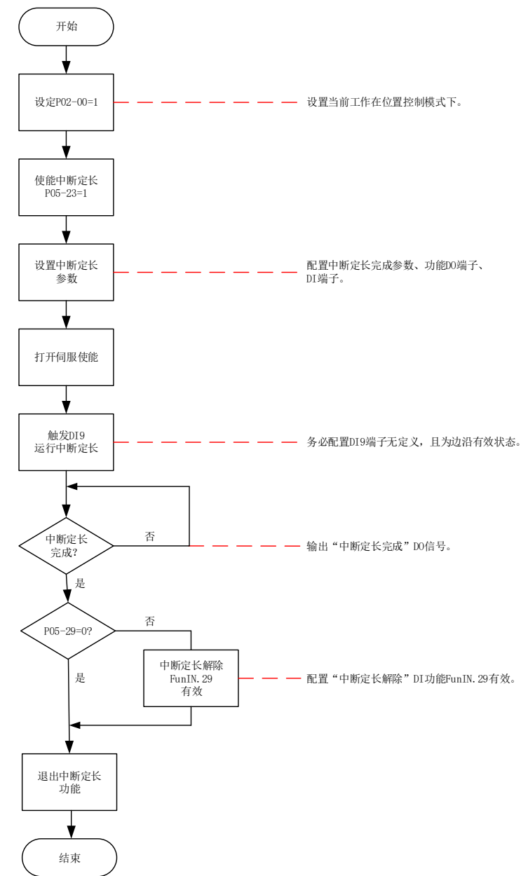
图 5-44 中断定长功能信号流程图
