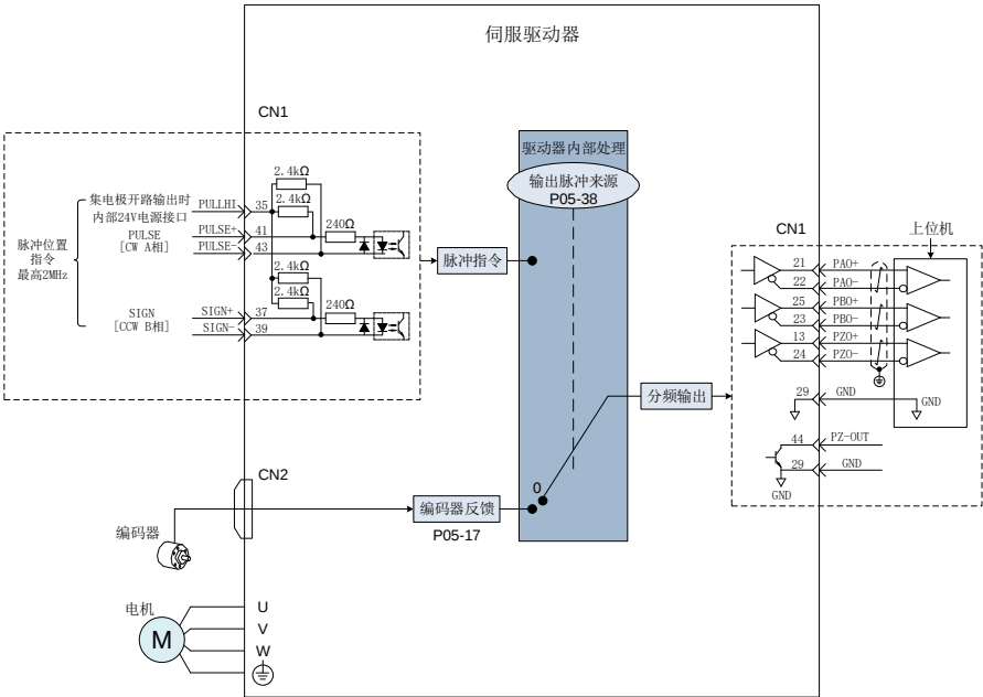
图 5-40 分频输出原理示意图
