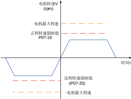
图 5-105 P07-17=0 速度限制曲线图
