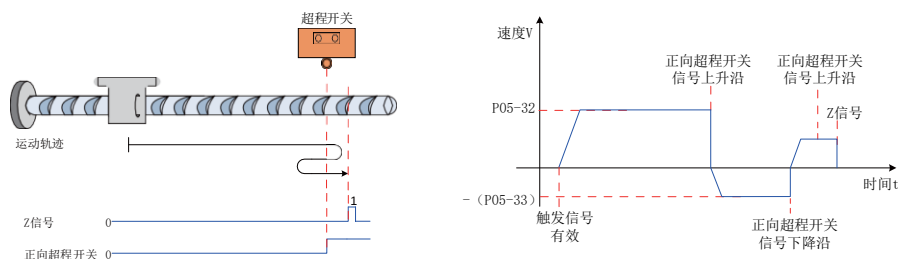
图 5-57 模式 8 原点回零电机运行曲线①与转速说明
