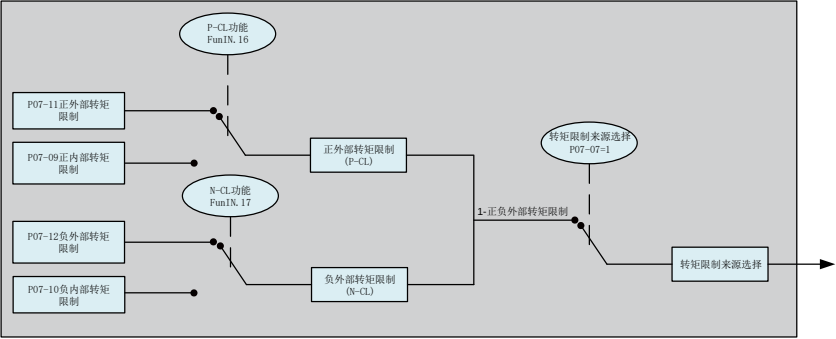
图 5-98 P07-07=1 转矩限制来源
