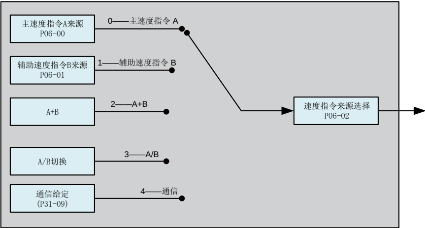
图 5-65 速度指令来源图
