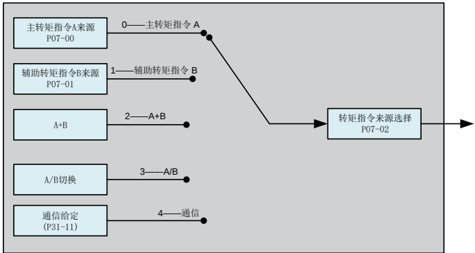
图 5-85 转矩指令来源图
