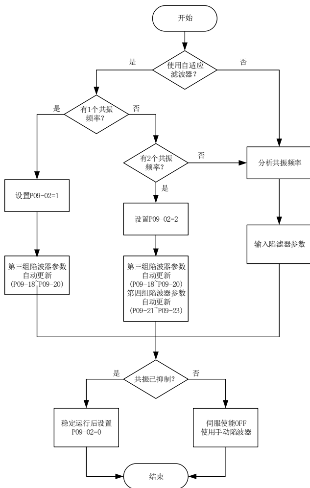
图 6-14 陷波器使用步骤
