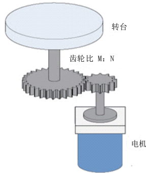
图 5-111 旋转负载示意图
