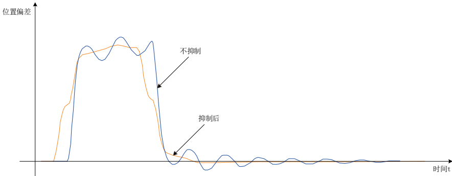
图 6-18 低频共振抑制效果图
