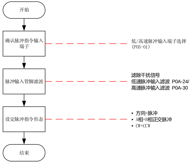
图 5-25 脉冲指令来源设置流程
