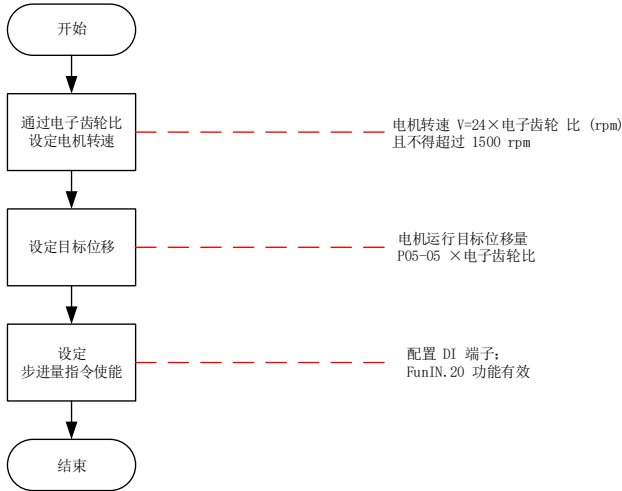
图 5-27 步进量指令来源设置流程
