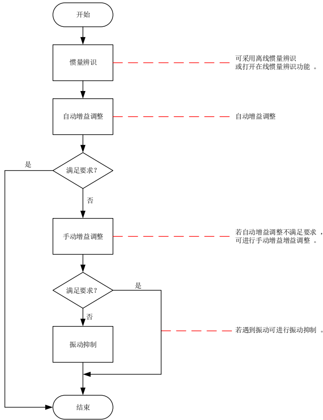
图 6-2 增益调整流程
