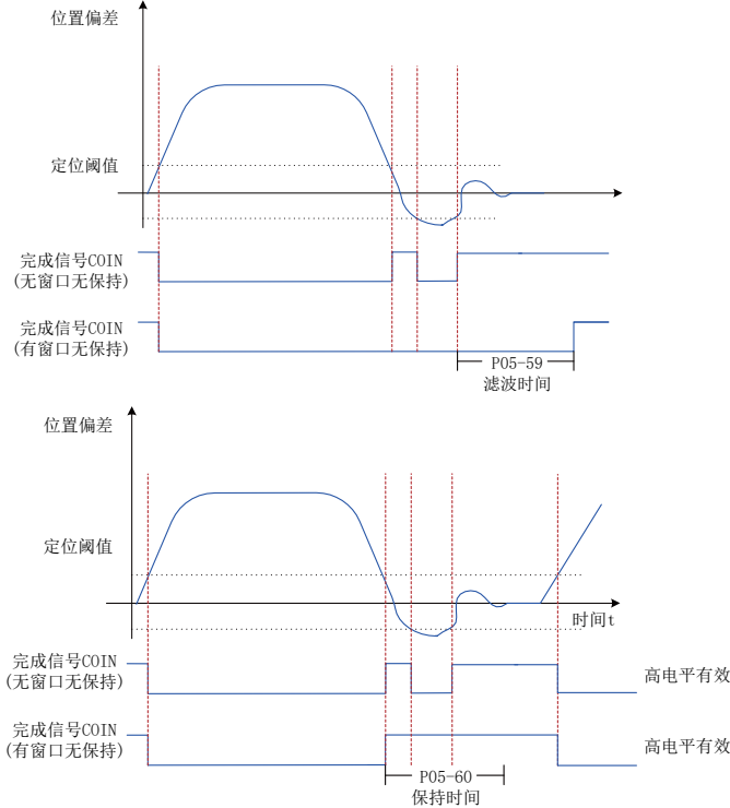
图 5-43 定位完成窗口时间和保持时间的原理图
