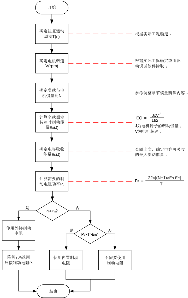
图 5-8 制动电阻选型流程图
