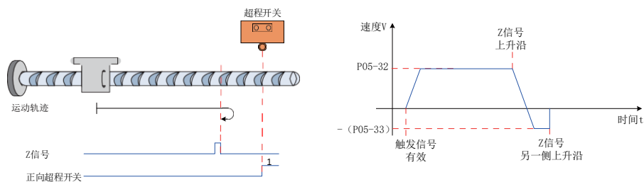
图 5-49 模式 2 原点回零电机运行曲线①与转速说明
