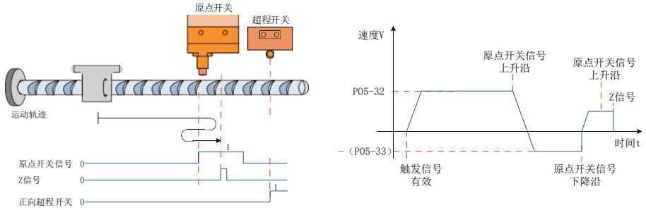
图 5-52 模式 4 原点回零电机运行曲线①与转速说明
