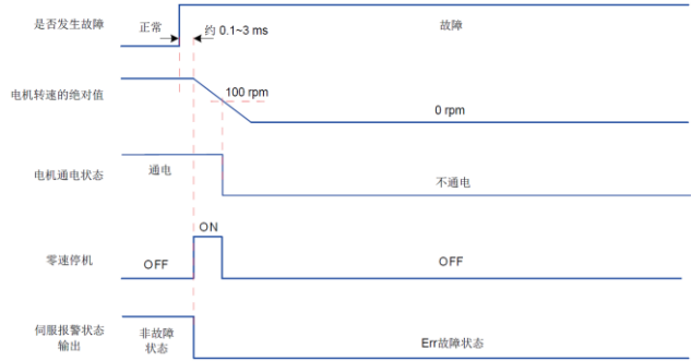
图 5-15 故障 2 (非抱闸) 时零速停机保持自由运行状态时序图
