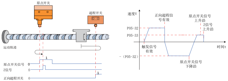
图 5-54 模式 4 原点回零电机运行曲线③与转速说明
