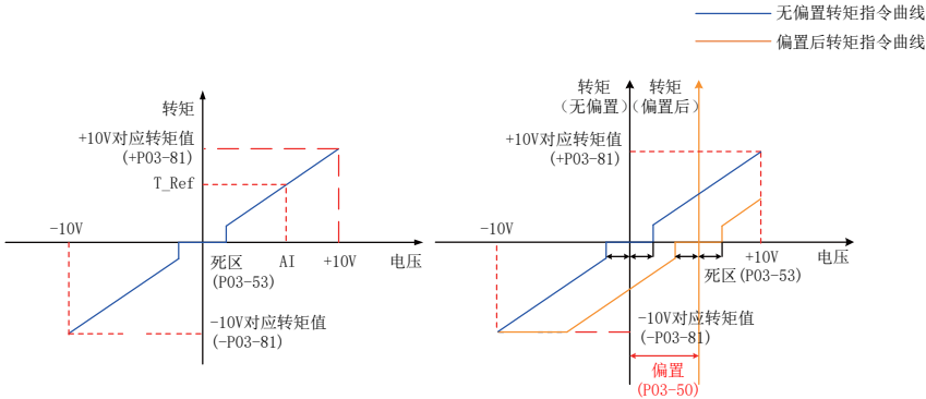
图 5-90 无偏置 AI2 示意图
