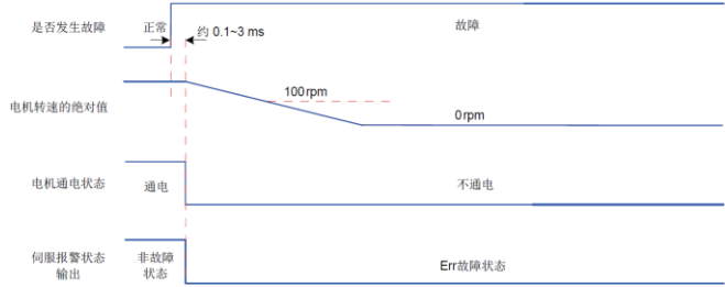
图 5-14 故障 2 时自由停机保持自由运行状态时序图
