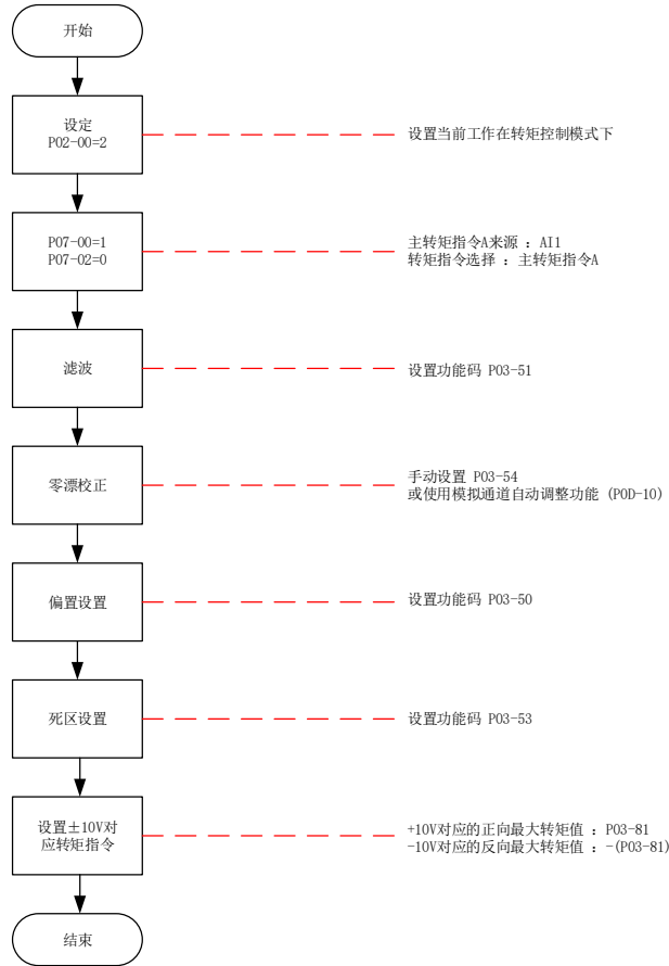
图 5-87 模拟量电压转矩指令操作流程
