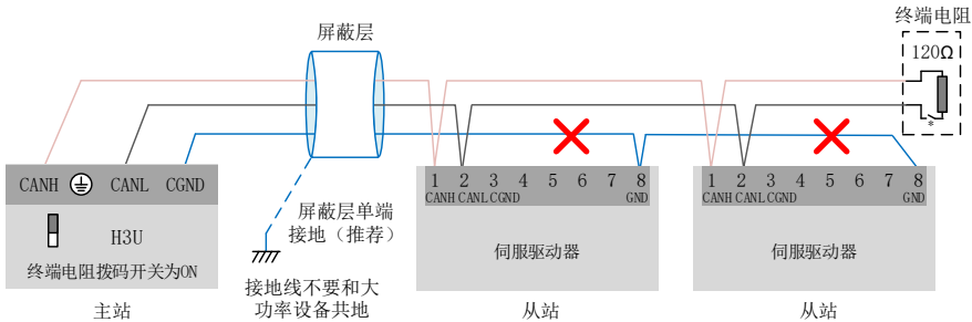
图 3-10 错误的 CAN 连接方法
