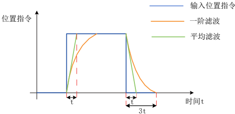
图 5-38 矩形位置指令一阶滤波与平均滤波示意图
