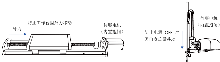
图 3-4 抱闸应用示意图
