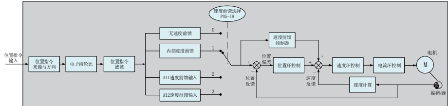
图 6-9 速度前馈控制操作图
