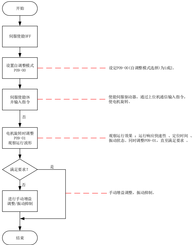
图 6-5 自动增益调整步骤
