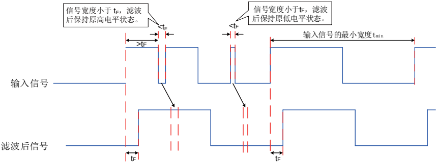
图 5-26 滤波信号波形举例
