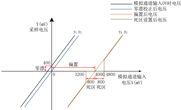
图 5-69 伺服驱动器 AI 处理对应采样电压举例
