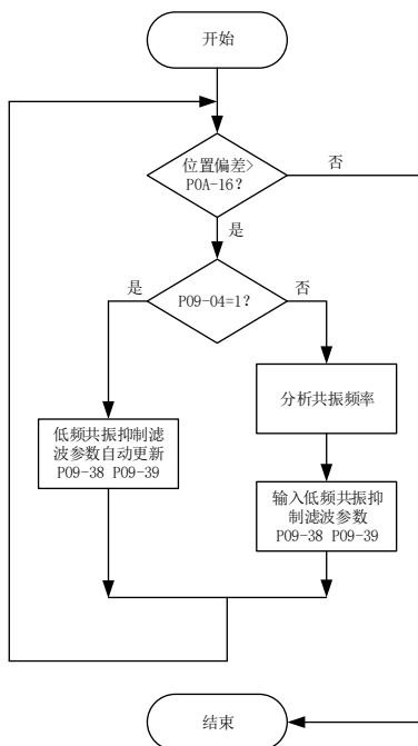
图 6-17 低频共振抑制滤波器使用步骤
