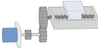
图 5-110 滚珠丝杠传动机构示意图
