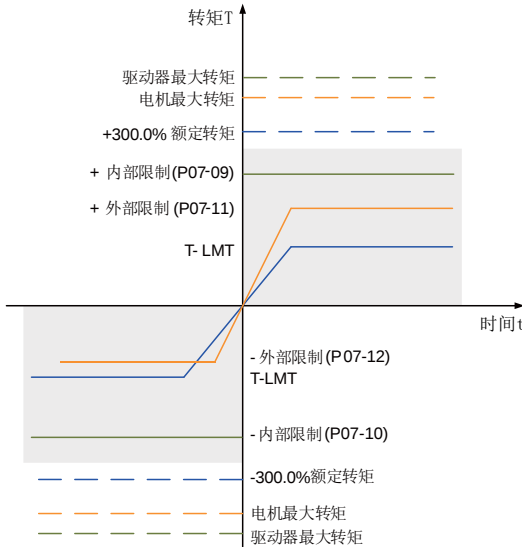
图 5-95 转矩限制举例
