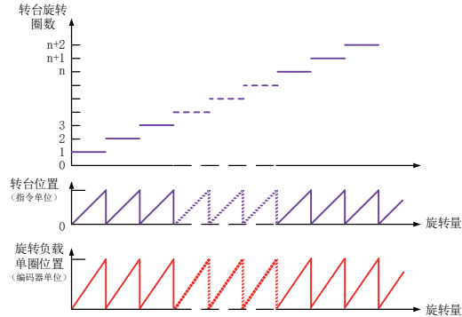
图 5-112 旋转负载单圈位置与转台位置对应关系示意图
