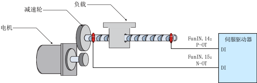
图 4-16 限位开关的安装示意图
