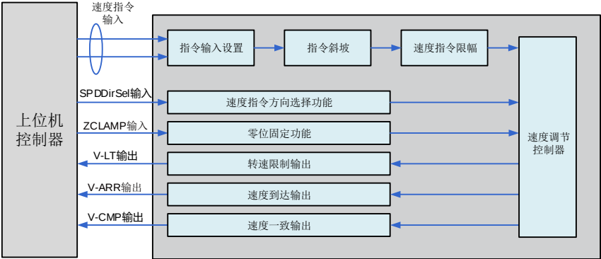
图 5-64 伺服驱动器与上位机信号交互图
