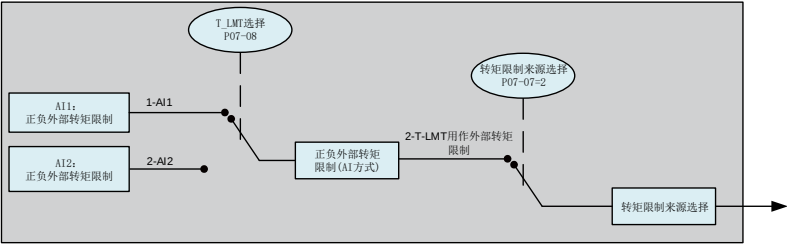
图 5-99 P07-07=2 转矩限制来源
