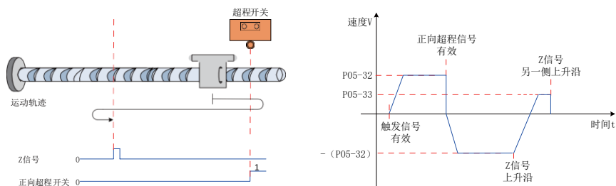
图 5-51 模式 2 原点回零电机运行曲线③与转速说明
