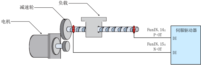
图 5-114 限位开关的安装示意图
