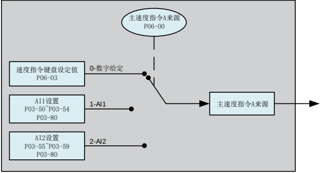
图 5-66 主速度指令 A 来源图
