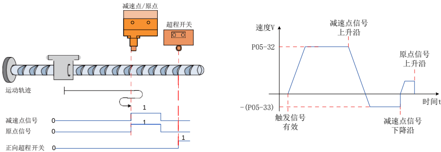
图 5-46 模式 0 原点回零电机运行曲线①与转速说明
