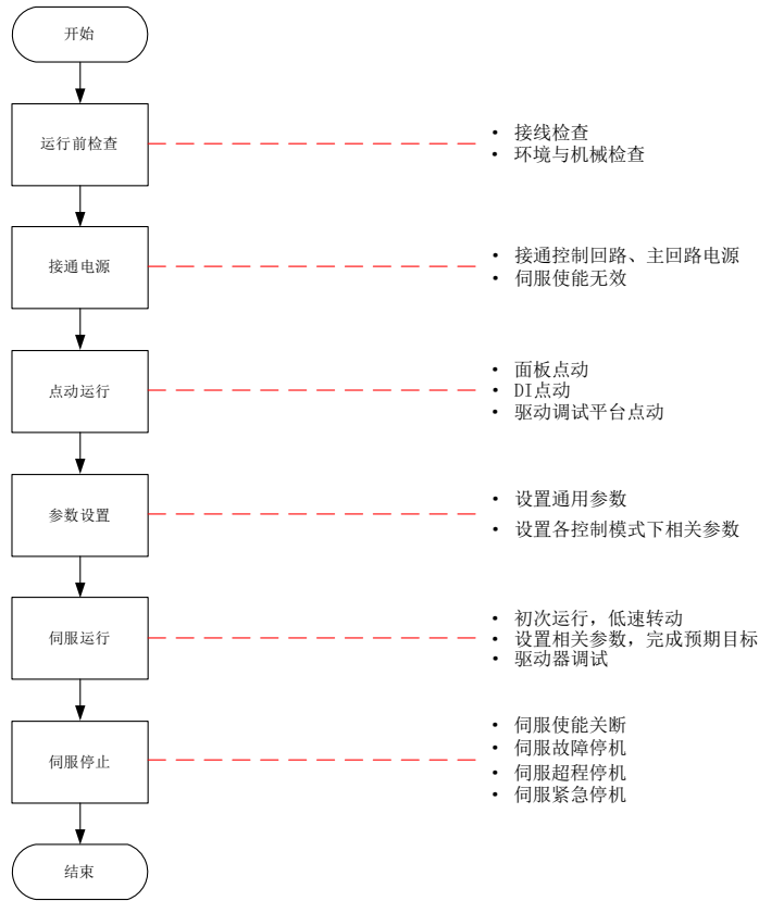
图 5-2 伺服设定流程
