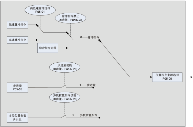
图 5-24 位置指令来源设置
