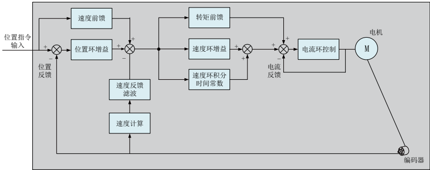
图 6-6 手动增益基本说明框图
