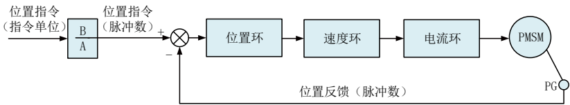
图 4-3 电子齿轮比作用原理图
