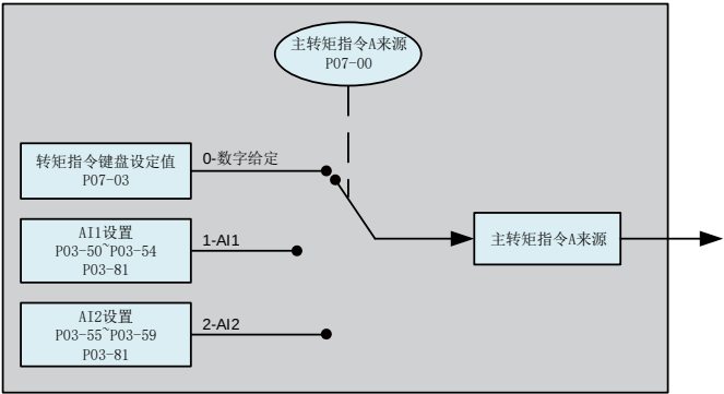
图 5-86 主转矩指令 A 来源说明
