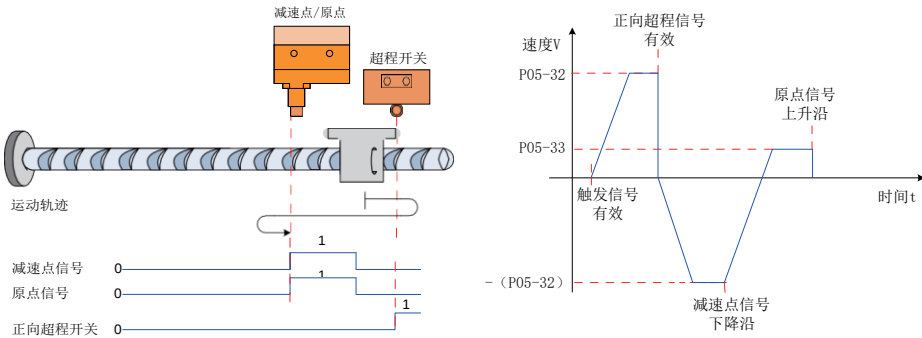
图 5-48 模式 0 原点回零电机运行曲线③与转速说明
