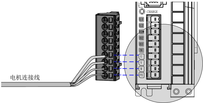
图 3-3 伺服驱动器输出与伺服电机连接举例
