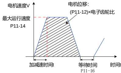
图 5-31 第 1 段电机运行曲线
