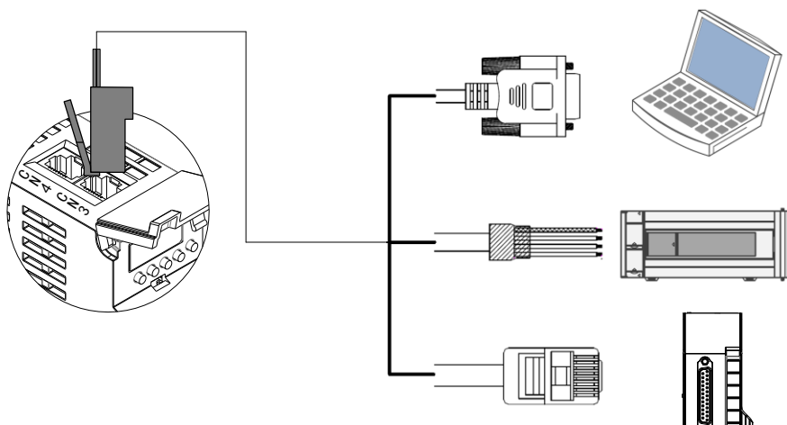
图 3-6 通信配线示意图
