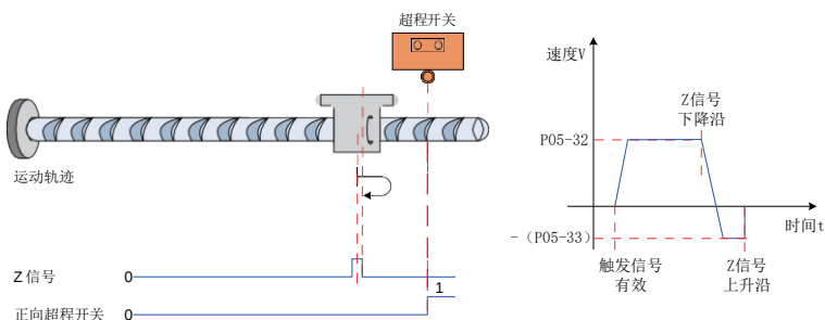
图 5-50 模式 2 原点回零电机运行曲线②与转速说明
