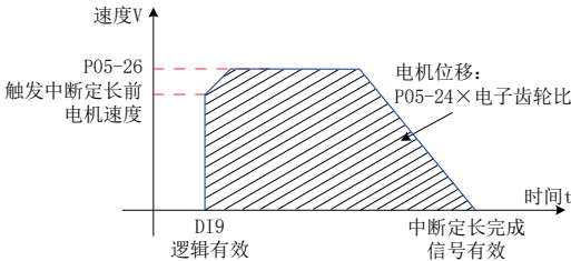
图 5-45 中断定长功能电机运行曲线
