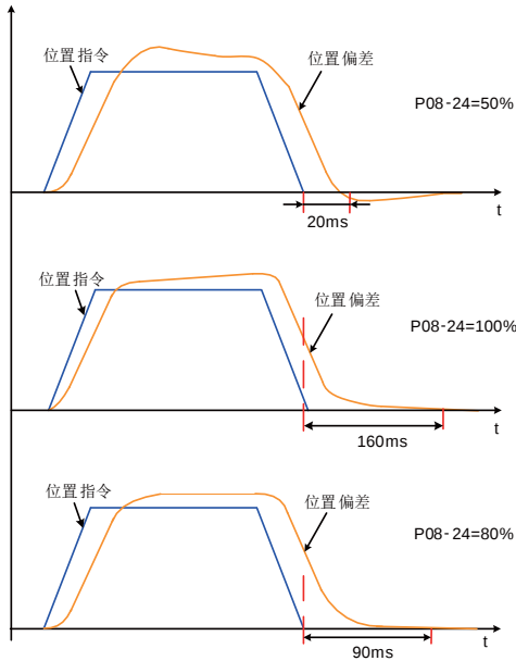
图 6-11 伪微分调节控制举例
