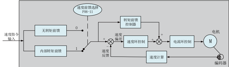
图 6-10 转矩前馈控制操作图
