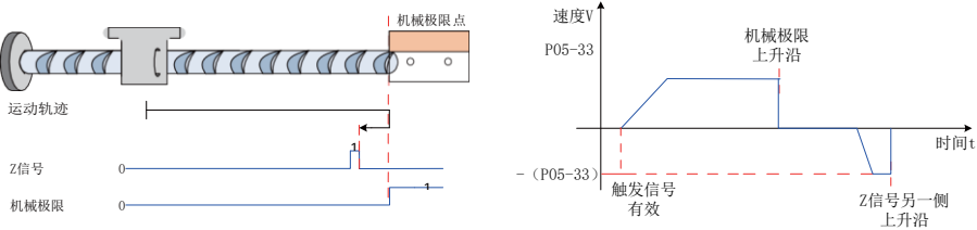
图 5-60 模式 12 原点回零电机运行曲线与转速说明
