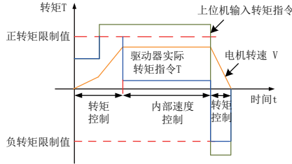
图 5-94 转矩给定与转矩限制
