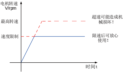
图 5-103 转矩模式速度限制示意图
