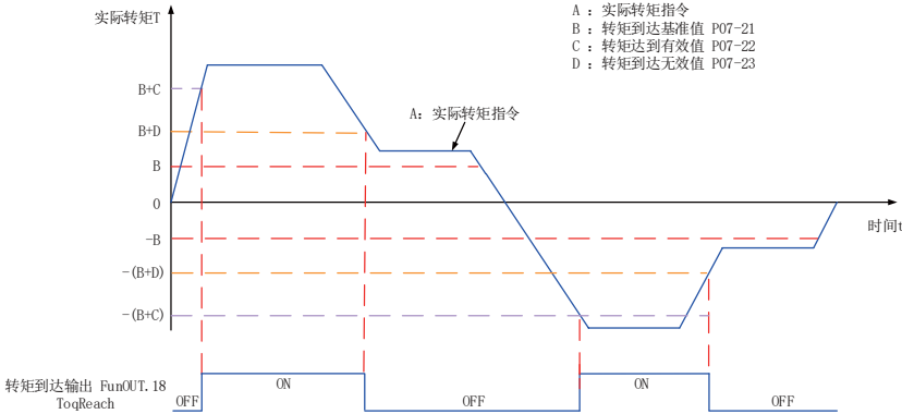
图 5-108 转矩到达输出波形举例
