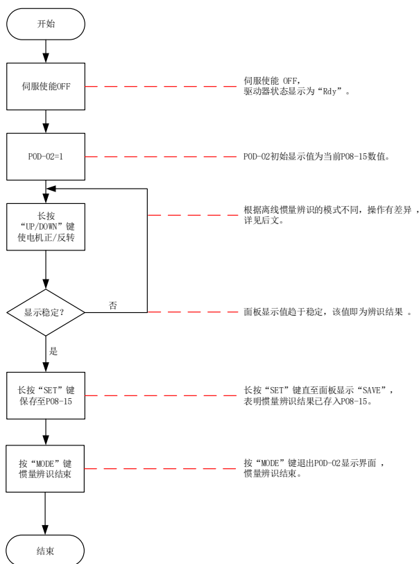
图 6-3 离线惯量辨识流程图
