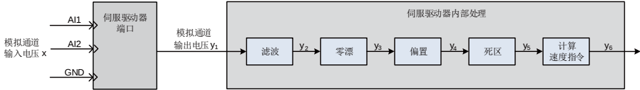
图 5-68 伺服驱动器 AI 处理流程
