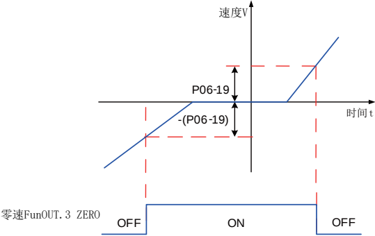
图 5-82 零速信号波形图
