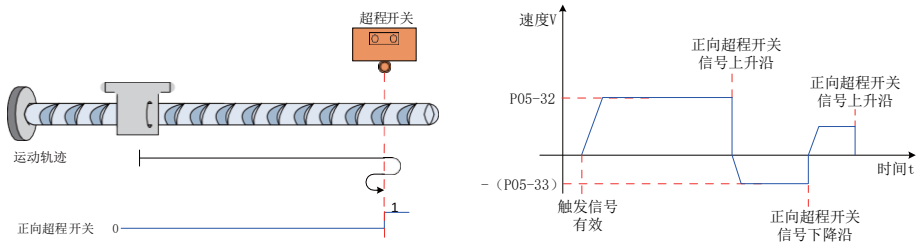
图 5-55 模式 6 原点回零电机运行曲线①与转速说明
