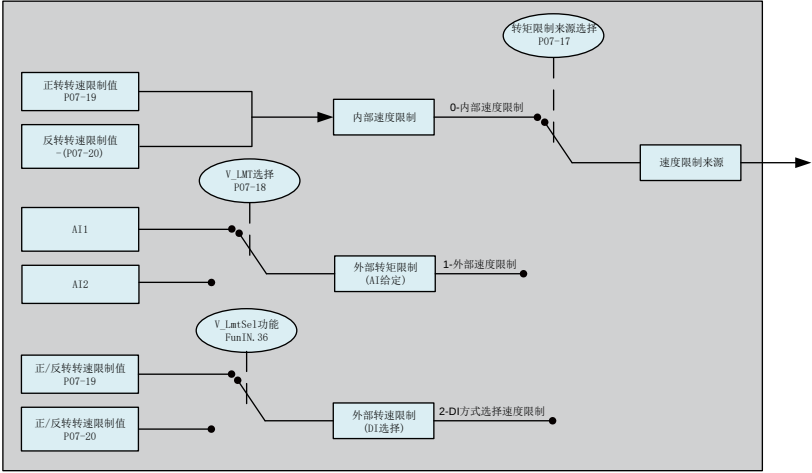
图 5-104 速度限制来源
