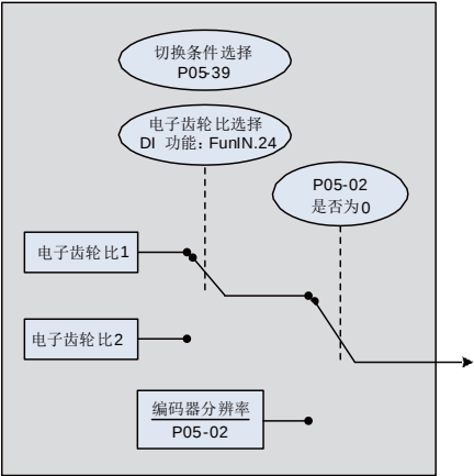
图 5-35 电子齿轮比设定操作流程
