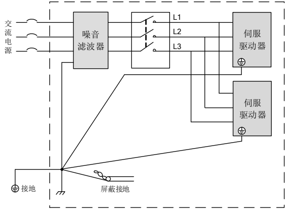
图 3-21 噪音滤波器地线处理示意图
