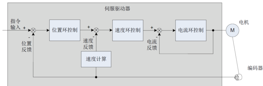
图 5-1 伺服系统控制简图
