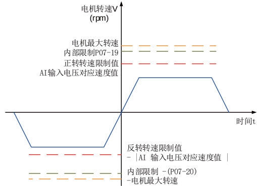
图 5-106 P07-17=1 速度限制曲线图
