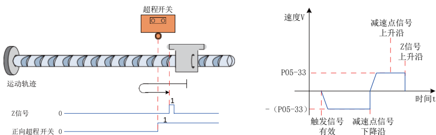
图 5-58 模式 8 原点回零电机运行曲线②与转速说明
