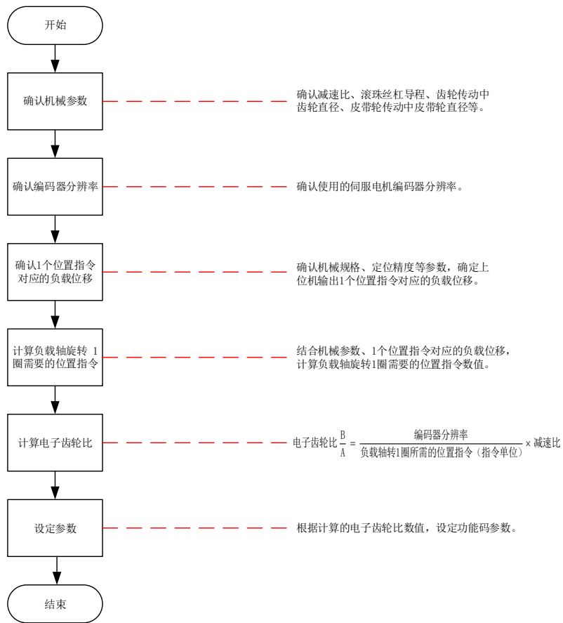
图 5-34 电子齿轮比设定步骤
