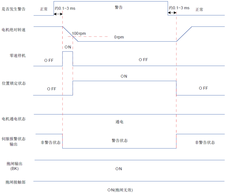
图 5-17 需停机类警告时序图
