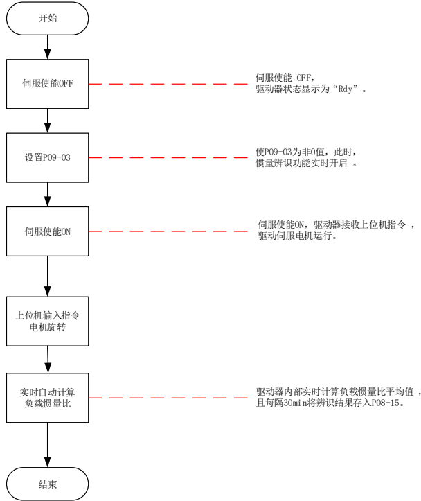
图 6-4 在线惯量辨识操作流程
