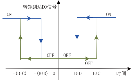
图 5-109 转矩到达输出有效说明
