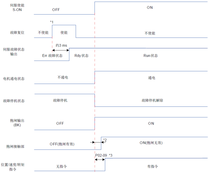
图 5-19 故障复位时序图
