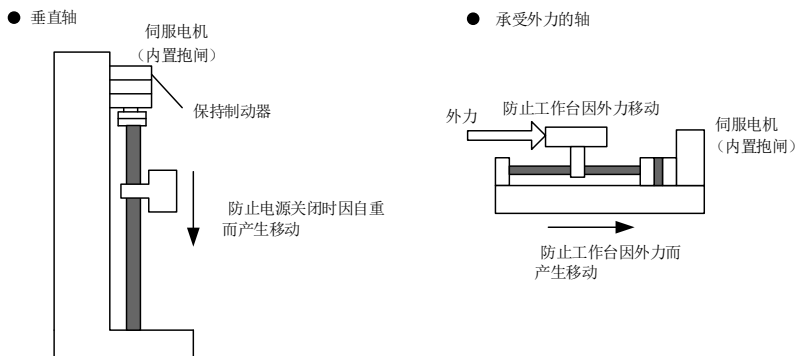
图 5-3 抱闸应用示意图
