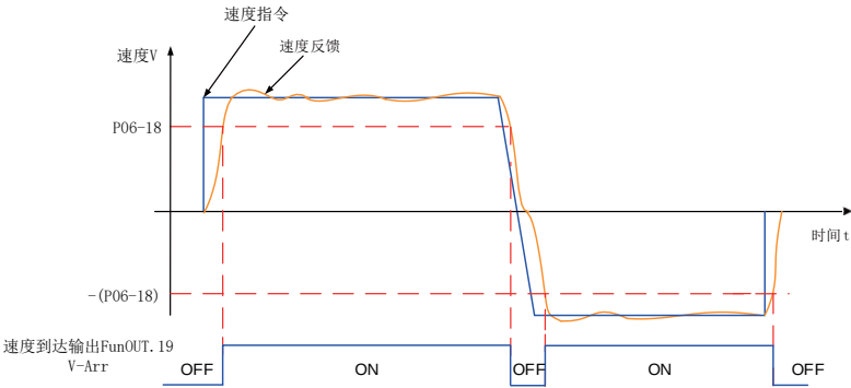
图 5-81 速度到达信号波形图
