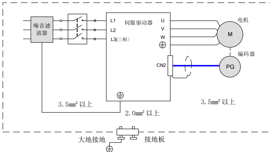
图 3-17 抗干扰配线实例
