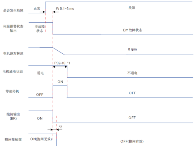
图 5-16 故障 2 (带抱闸) 时零速停机方式自由停机状态时序图
