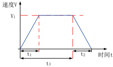
图 5-75 多段速度曲线举例
