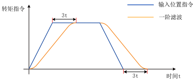
图 5-93 梯形转矩指令一阶滤波示意图
