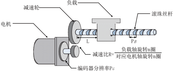
图 5-37 滚珠丝杠图示
