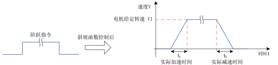
图 5-76 斜坡函数定义示意图
