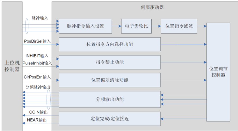
图 5-22 伺服驱动器与上位机信号交互图
