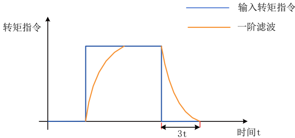
图 5-92 矩形转矩指令一阶滤波示意图
