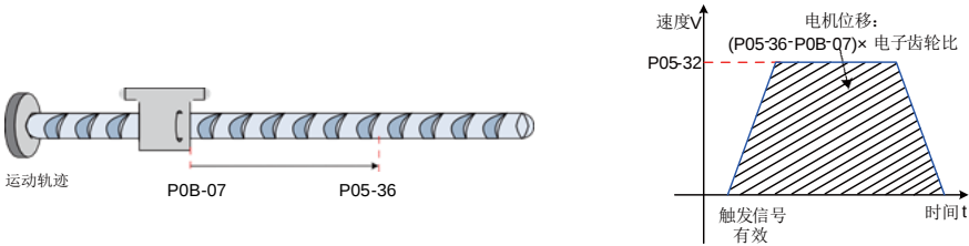
图 5-61 电气回零电机运行曲线与转速说明
