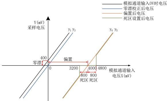
图 5-89 伺服驱动器 AI 处理对应采样电压举例
