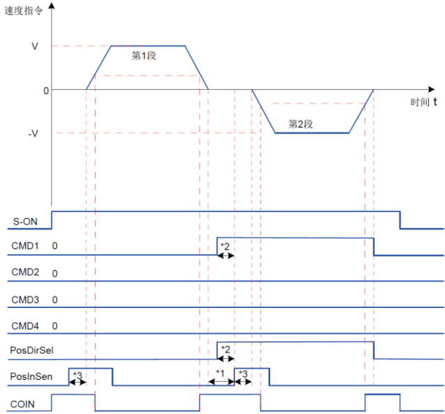
图 5-30 多段位置时序图
