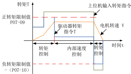
图 5-97 P07-07=0 转矩限制曲线图
