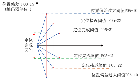
图 5-42 位置偏差相关信号
