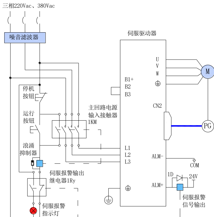
图 3-2 三相 220V 主电路配线
