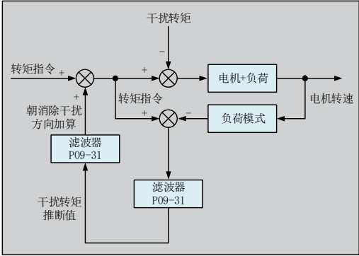
图 6-12 扰动观测功能框图
