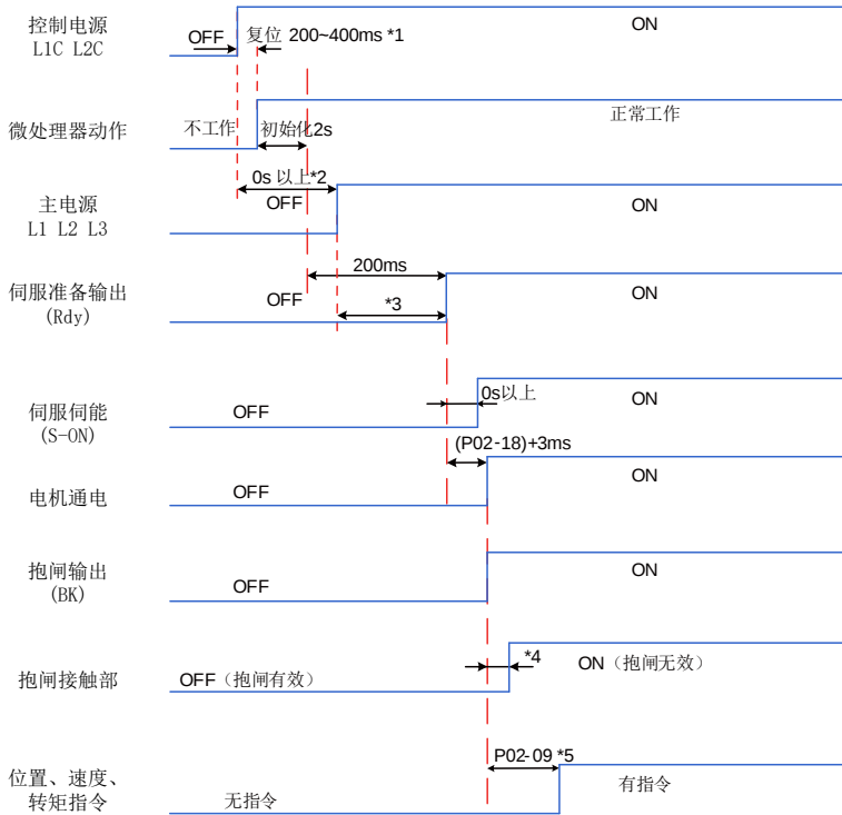
图 5-12 电源接通时序图
