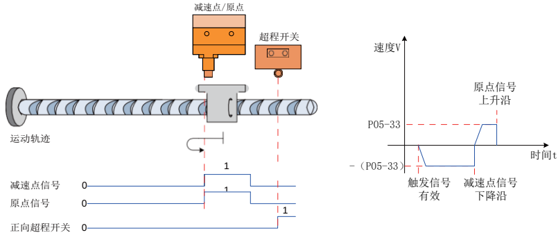
图 5-47 模式 0 原点回零电机运行曲线②与转速说明
