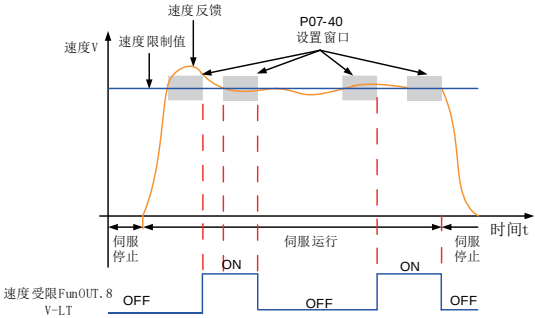
图 5-107 速度限制 DO 输出波形举例
