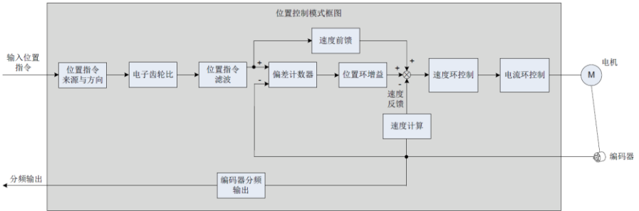
图 5-21 位置控制框图
