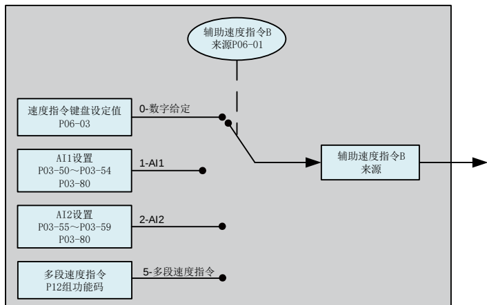
图 5-72 辅助速度指令 B 来源图
