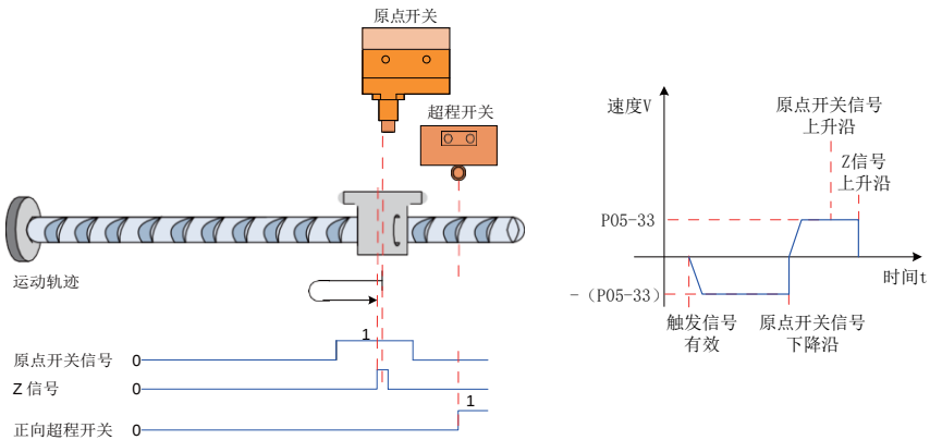
图 5-53 模式 4 原点回零电机运行曲线②与转速说明
