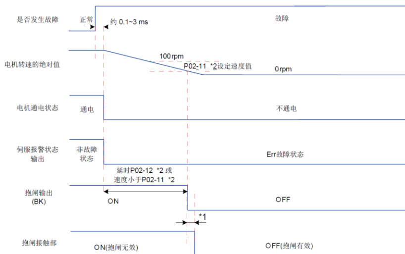
图 5-13 故障 1 时自由停机保持自由运行状态时序图
