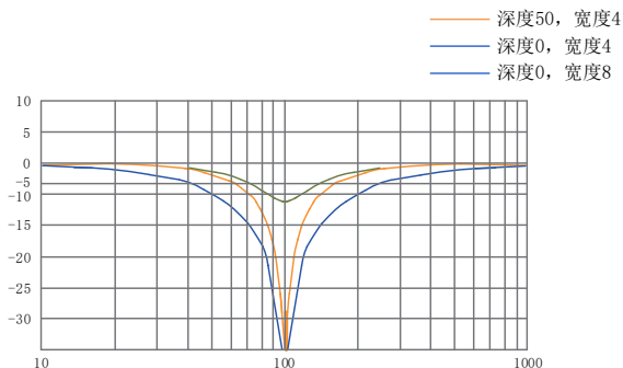
图 6-15 陷波器频率特性
