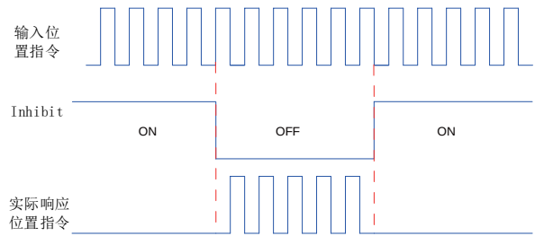
图 5-32 位置指令禁止功能波形举例
