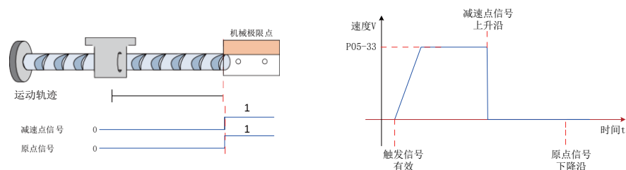
图 5-59 模式 10 原点回零电机运行曲线与转速说明
