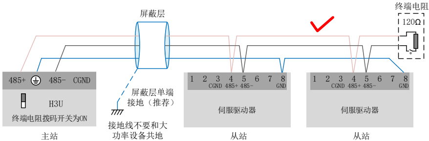
图 3-13 正确的 485 连接方法
