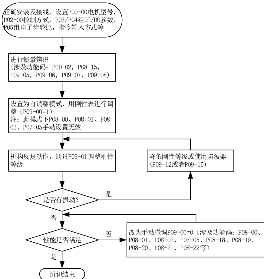
图 4-17 一般调试流程图
