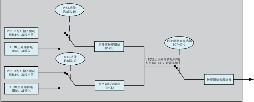
图 5-101 P07-07=3 转矩限制来源
