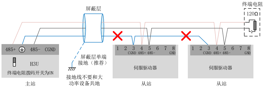
图 3-14 错误的 485 连接方法
