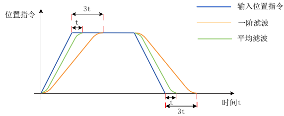
图 5-39 梯形位置指令一阶滤波与平均滤波示意图
