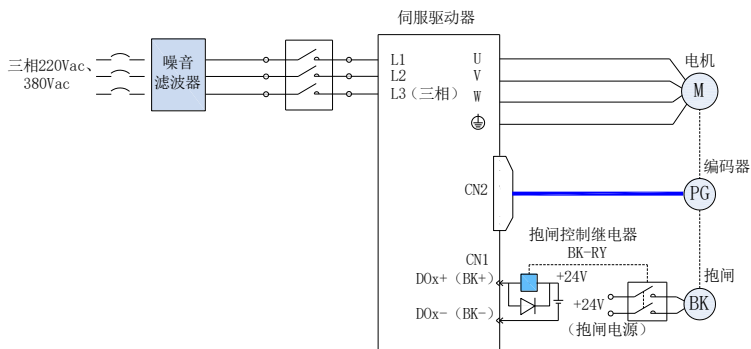
图 3-5 抱闸配线图
