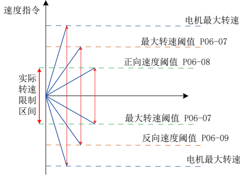
图 5-78 速度指令限幅举例说明
