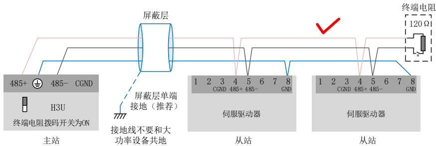
图 3-11 正确的 485 连接方法
