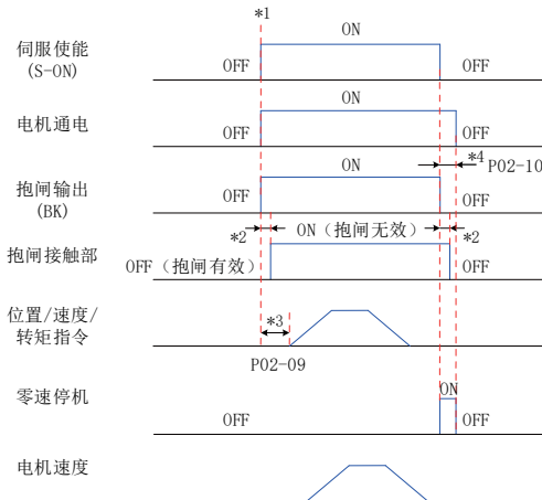
图 5-5 电机静止时抱闸时序图
