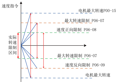
图 4-9 速度指令限幅举例说明图
