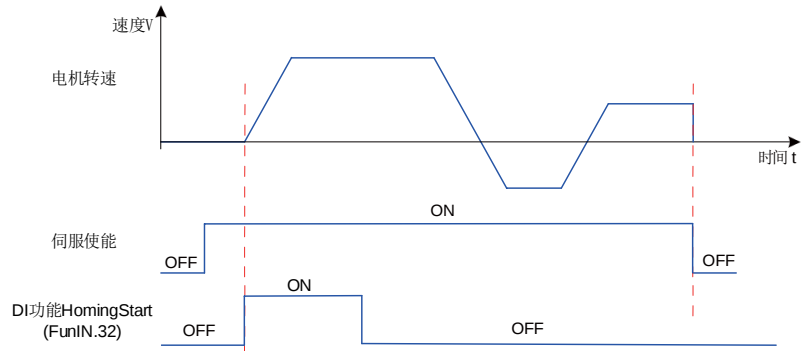
图 5-62 时序图举例
