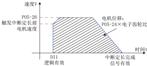
图 5-45 中断定长功能电机运行曲线
