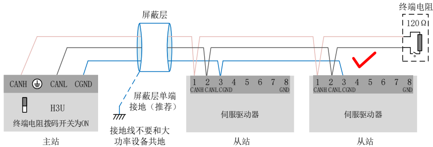
图 3-7 正确的 CAN 连接方法
