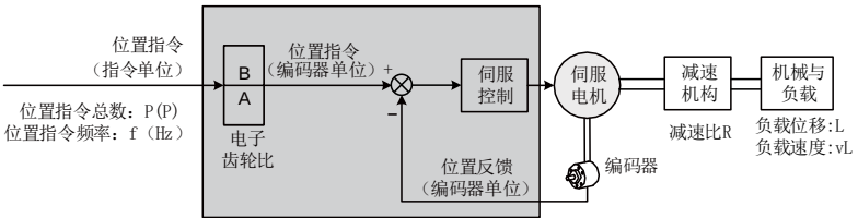
图 5-36 位置指令 (指令单位)、负载位移与电子齿轮比之间的关系
