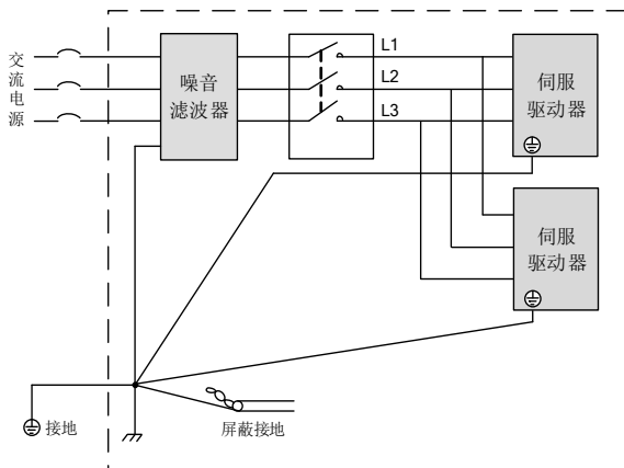
图 3-21 噪音滤波器地线处理示意图
