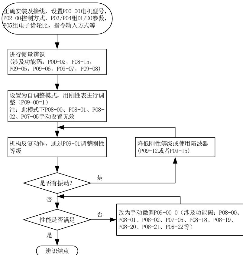
图 4-17 一般调试流程图
