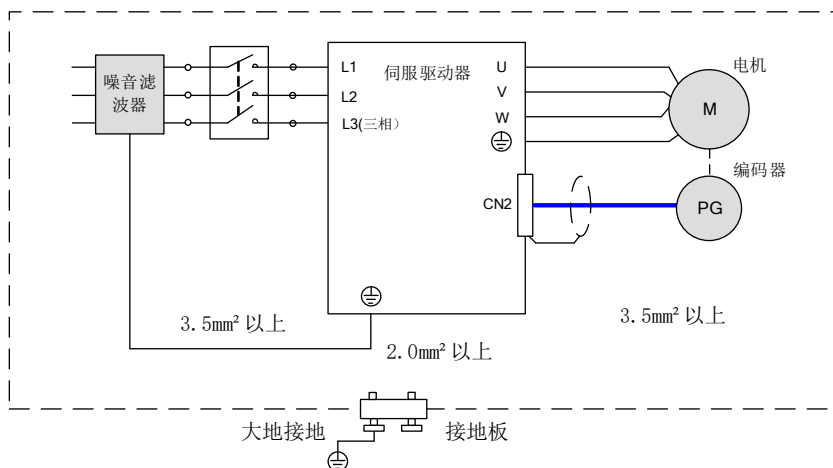
图 3-17 抗干扰配线实例
