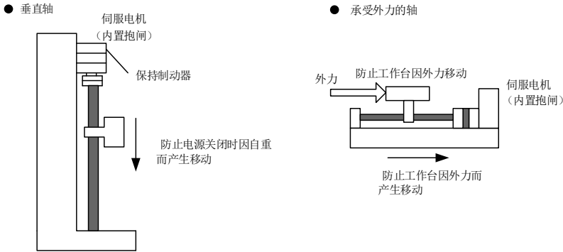
图 5-3 抱闸应用示意图
