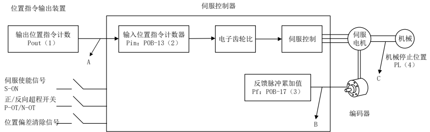
图 10-1 定位控制原理框图
