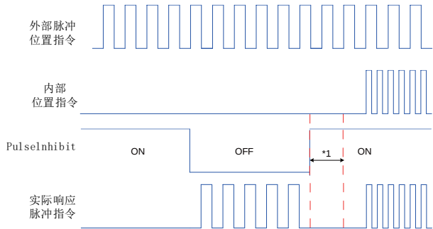
图 5-33 脉冲指令禁止功能波形举例
