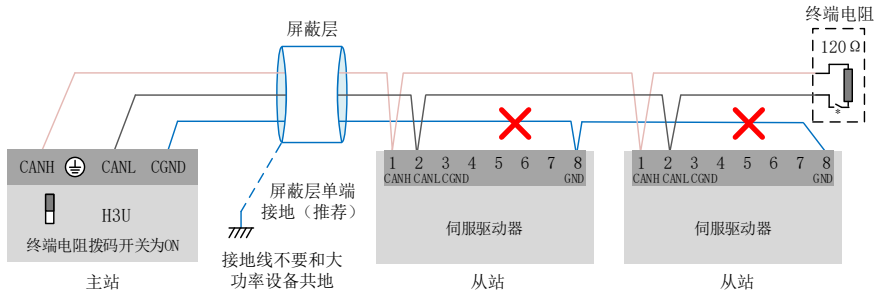
图 3-8 错误的 CAN 连接方法
