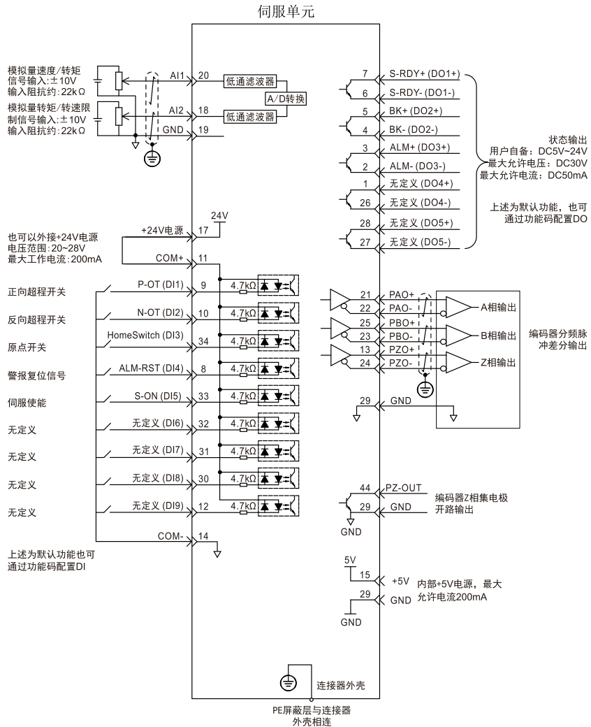
图 4-11 转矩模式配线图
