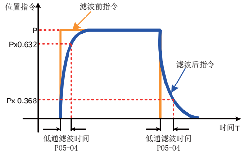
图 4-4 一阶滤波示例图
