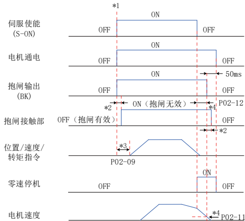
图 5-6 电机旋转时抱闸时序图
