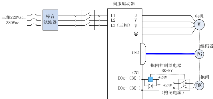
图 5-4 抱闸配线图
