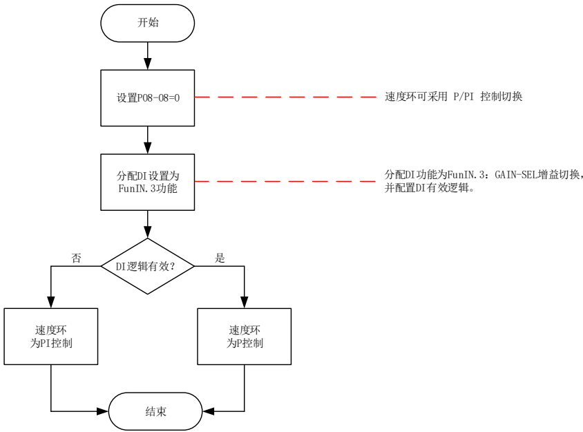
图 6-7 P08-08=0 增益切换流程图
