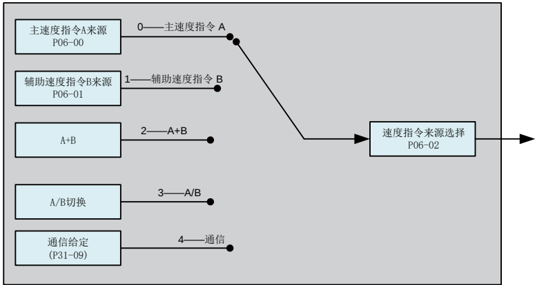
图 5-65 速度指令来源图
