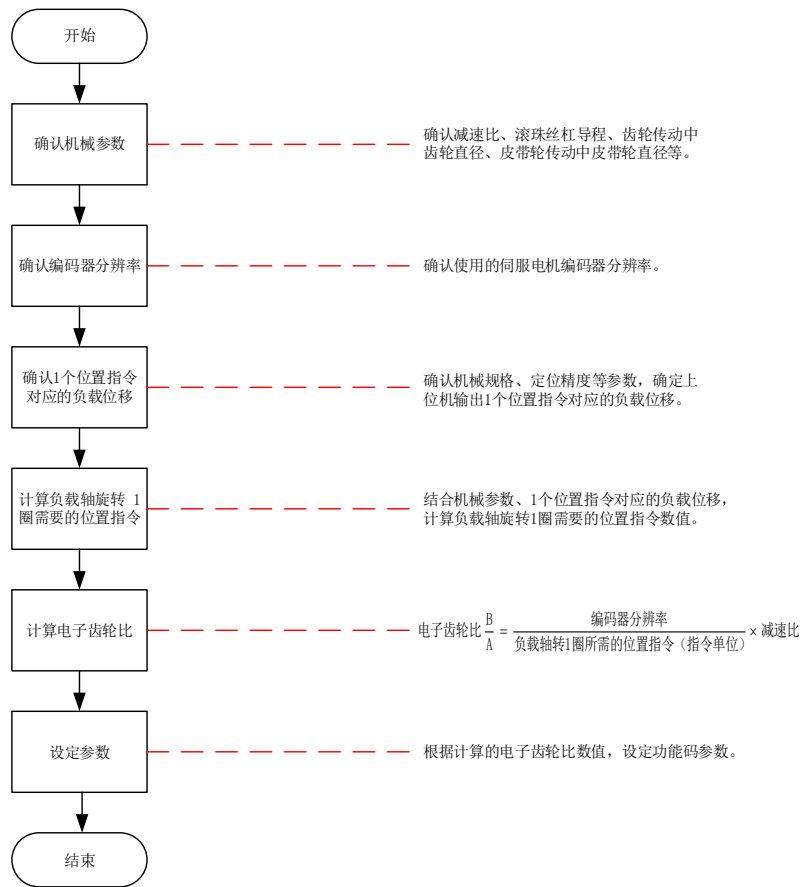
图 5-34 电子齿轮比设定步骤
