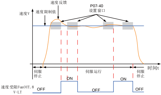
图 5-107 速度限制 D0 输出波形举例
