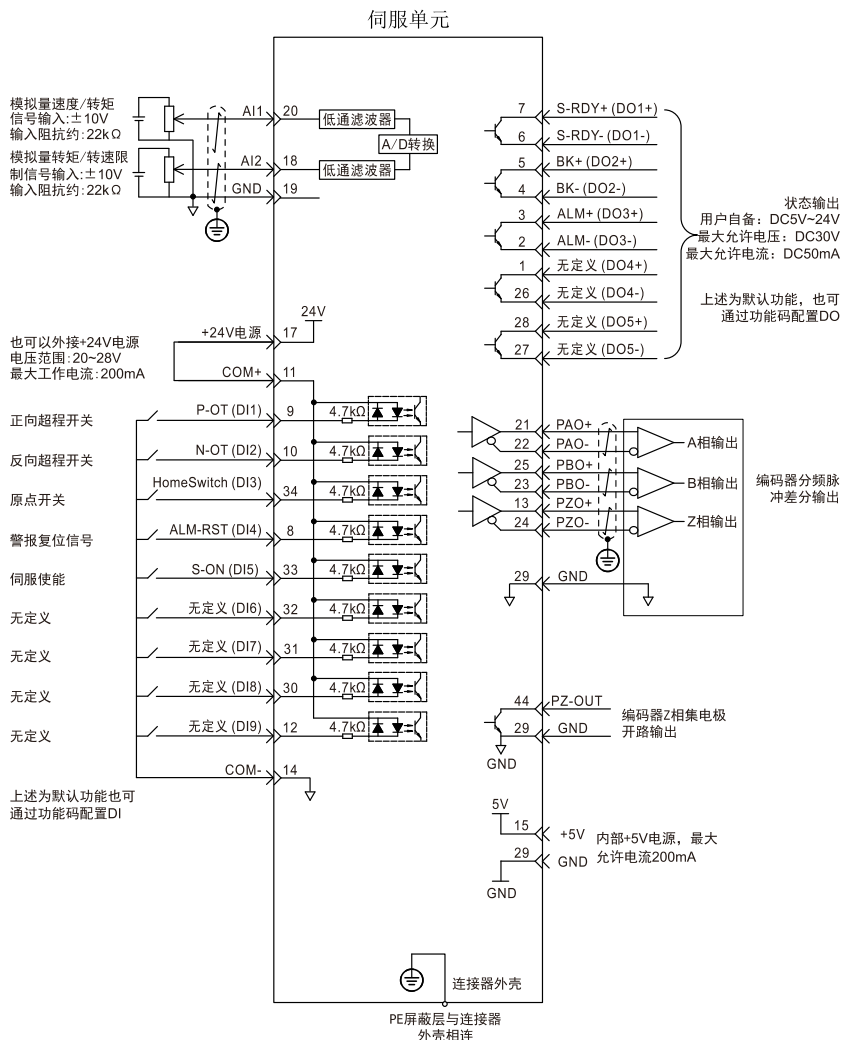
图 4-6 速度模式配线图
