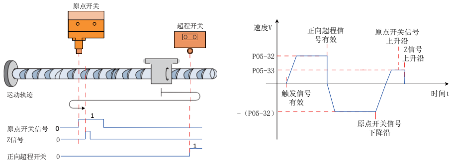
图 5-54 模式 4 原点回零电机运行曲线③与转速说明
