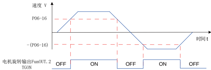
图 5-79 电机旋转信号波形图
