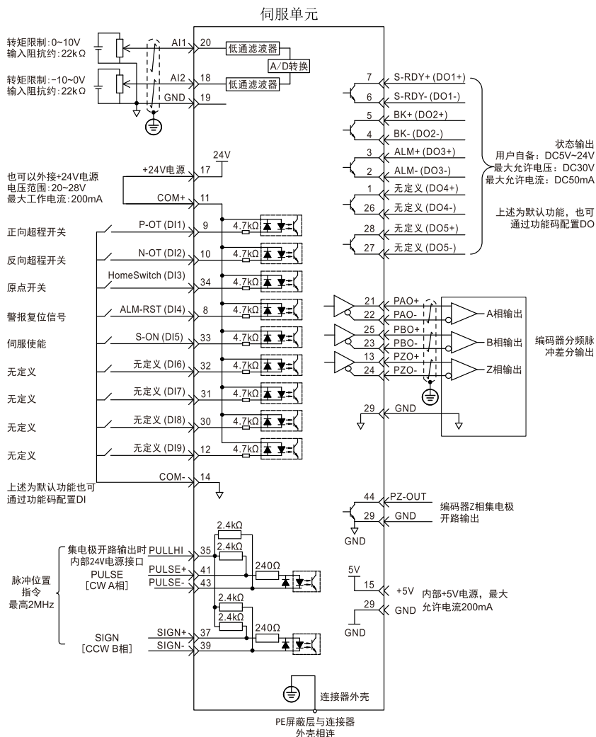
图 4-2 位置模式配线图
