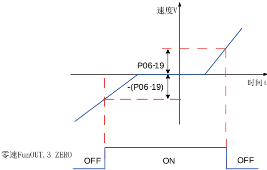
图 5-82 零速信号波形图
