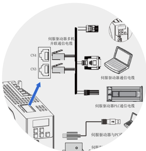
图 3-4 通信配线示意图
