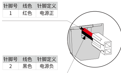
图 3-16 绝对值编码器电池外引线说明
