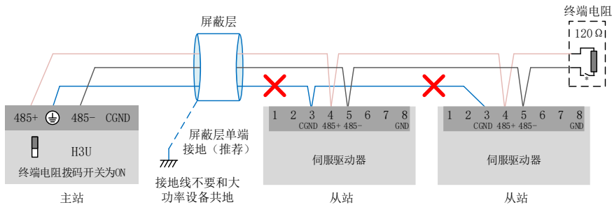
图 3-12 错误的 485 连接方法
