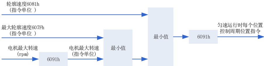
图 9-6 轮廓速度 6081h-速度限制
