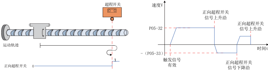
图 6-45 模式 6 原点回零电机运行曲线①与转速说明
