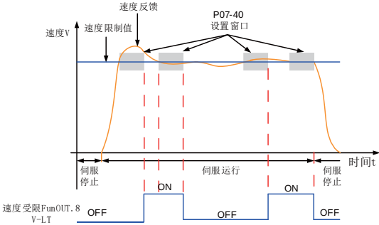
图 6-79 速度限制 DO 输出波形举例
