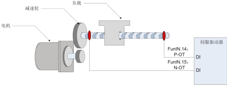
图 6-7 限位开关的安装示意图
