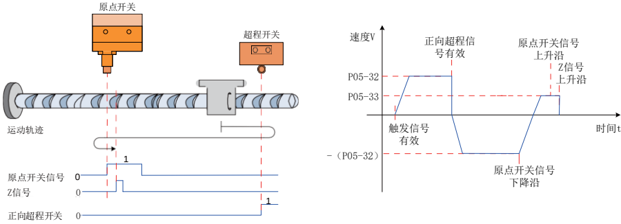
图 6-44 模式 4 原点回零电机运行曲线③与转速说明
