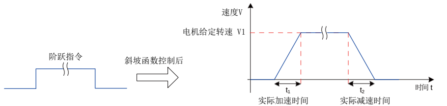
图 6-61 斜坡函数定义示意图
