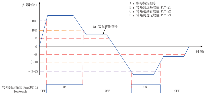
图 6-80 转矩到达输出波形举例
