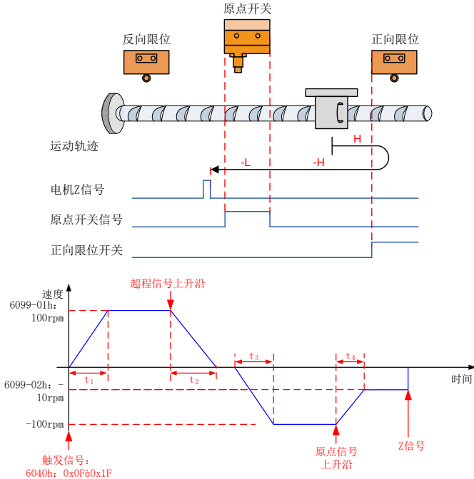
图 9-30 6098=7 且减速点信号无效, 遇到限位开关模式②
