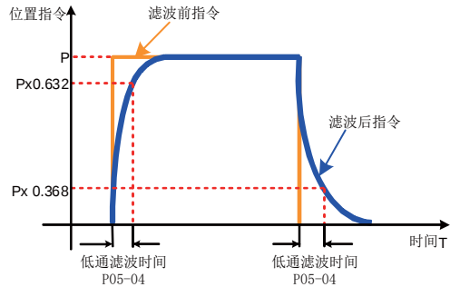
图 5-3 一阶滤波示例图
