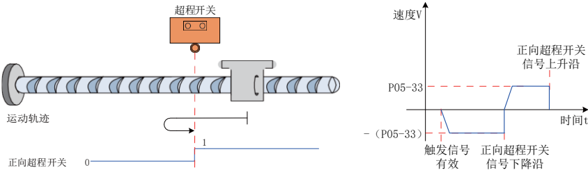
图 6-46 模式 6 原点回零电机运行曲线②与转速说明
