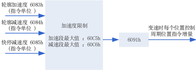
图 9-7 轮廓加速度限制
