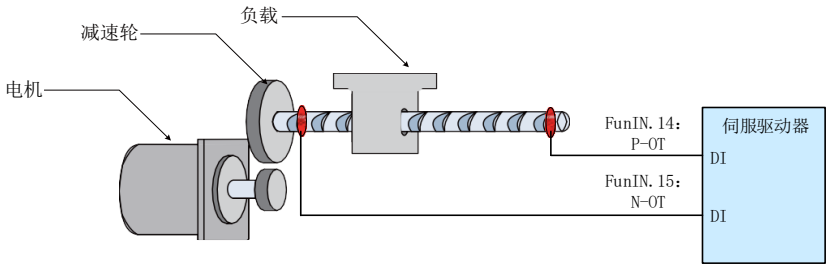
图 5-13 限位开关的安装示意图
