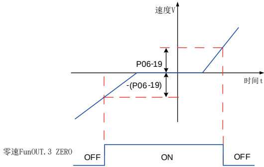
图 6-67 零速信号波形图
