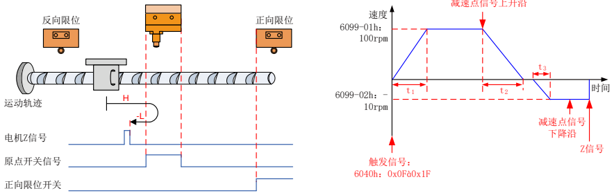
图 9-29 6098=7 且减速点信号无效, 未遇到限位开关模式①
