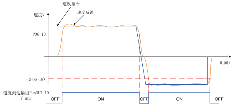
图 6-66 速度到达信号波形图
