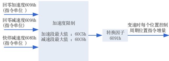
图 9-16 回零加速度 609Ah 限制
