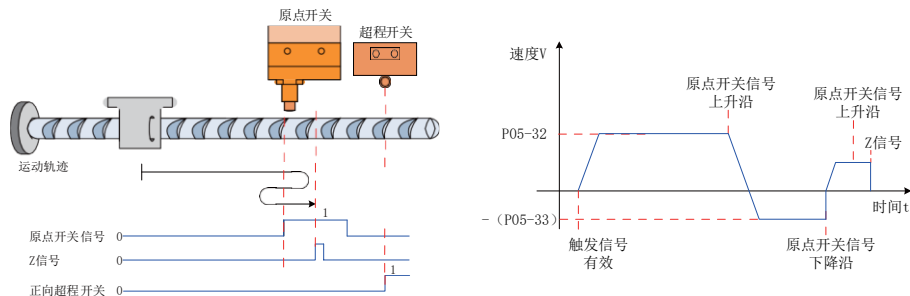
图 6-42 模式 4 原点回零电机运行曲线①与转速说明
