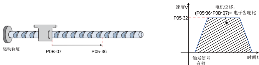
图 6-51 电气回零电机运行曲线与转速说明
