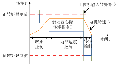
图 6-74 转矩给定与转矩限制
