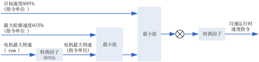
图 9-52 目标速度 60FFh-速度限制
