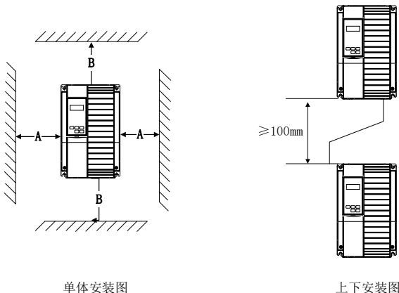
图 3-1 安装示意图
