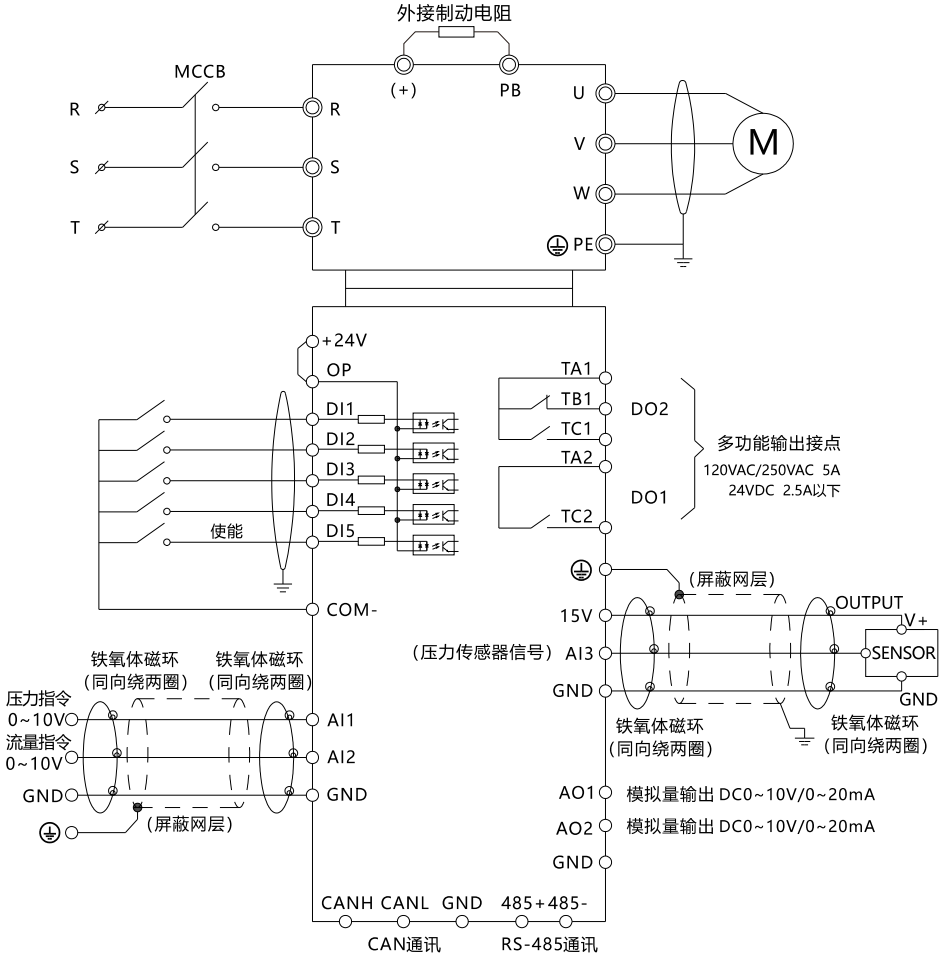
图 3-3 标准接线图
