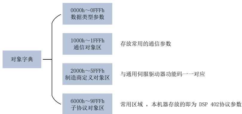
图 7-1 CANopen 对象字典结构说明图
