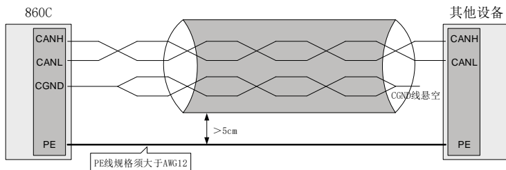
图 2-15 其它设备 CAN 无外接地端口
