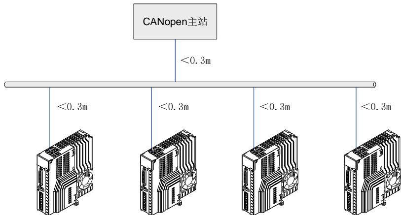
图 2-4 CAN 通信网络拓扑结构
