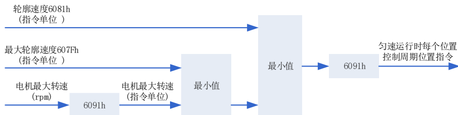
图 4-6 轮廓速度 6081h-速度限制
