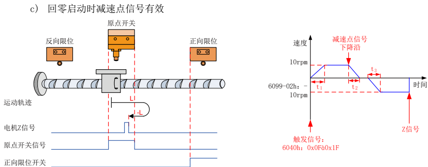
图 4-37 6098h=9 且减速点信号有效模式③
