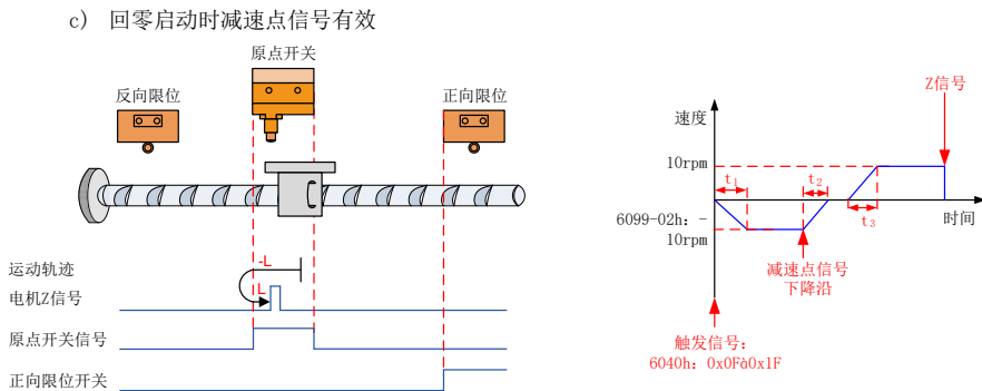
图 4-34 6098h=8 且减速点信号有效模式③
