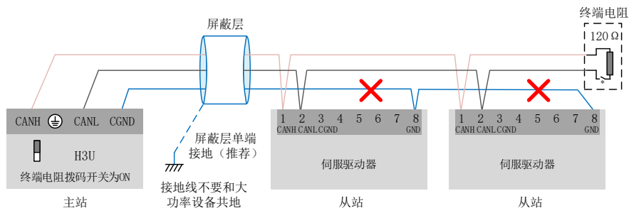
图 2-13 错误的 CAN 连接方法
