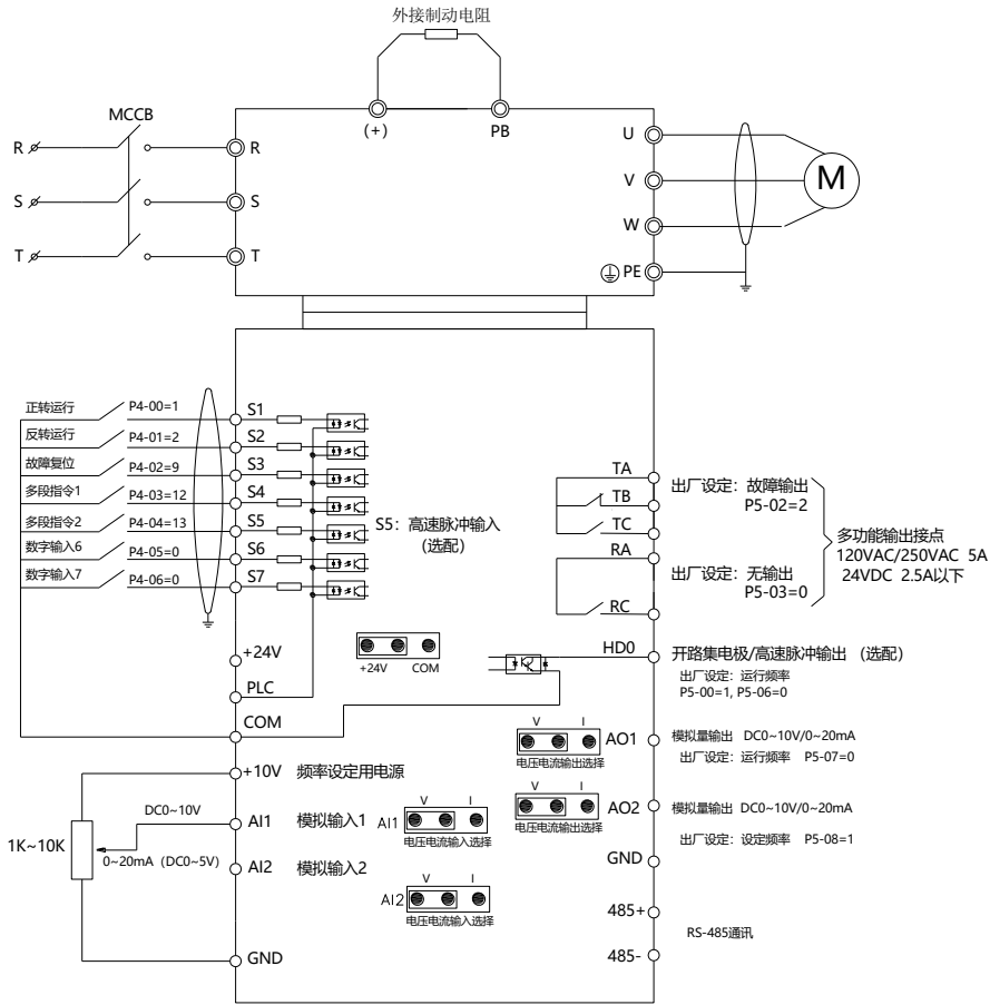
图 3-4 标准接线图
