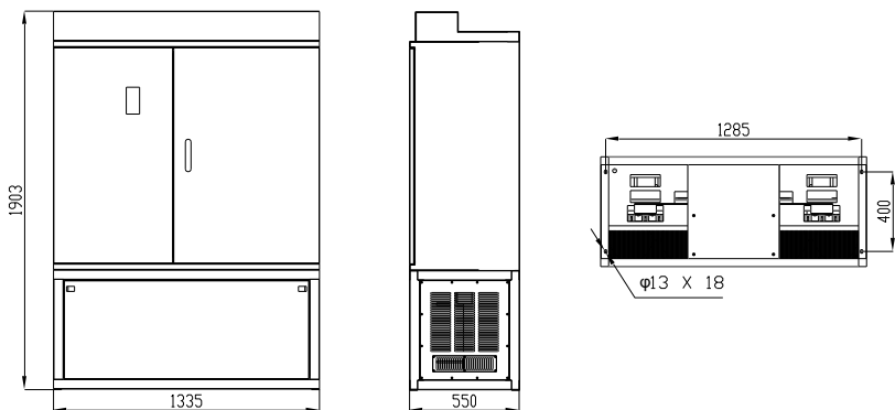
图 2-8 9000G~14000G 落地安装示意图
