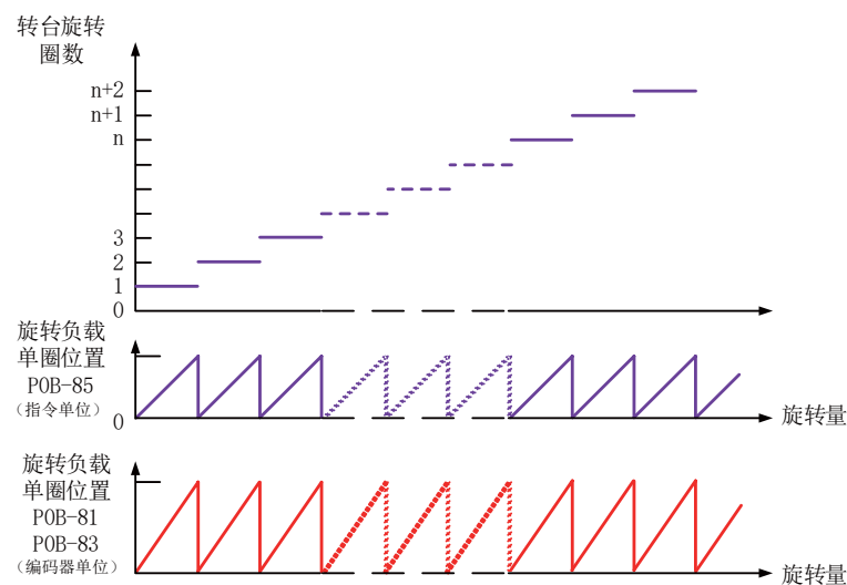
图 7-41 旋转负载单圈位置与转台位置对应关系示意图
