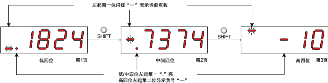
图 5-3 -1073741824 显示操作示意图
