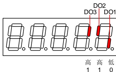
图 5-14 D0 端子电平均为“高电平有效”时 P0B-05 显示
