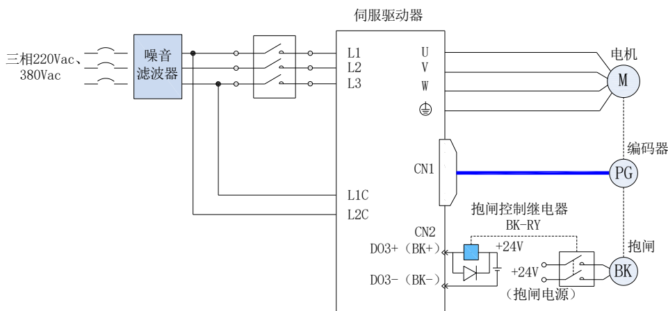
图4-10 抱闸配线图
