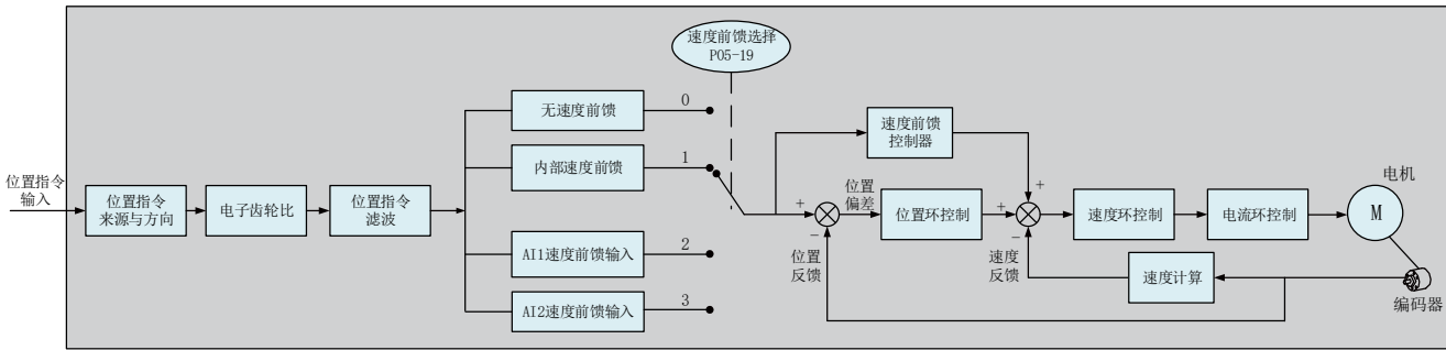
图 9-9 速度前馈控制操作图
