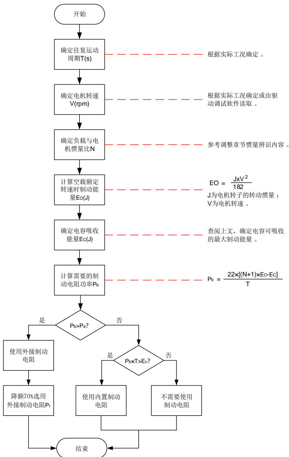
图7-8 制动电阻选型流程图
