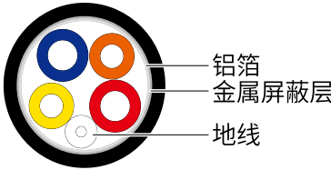
图4-9 推荐线缆示意图
