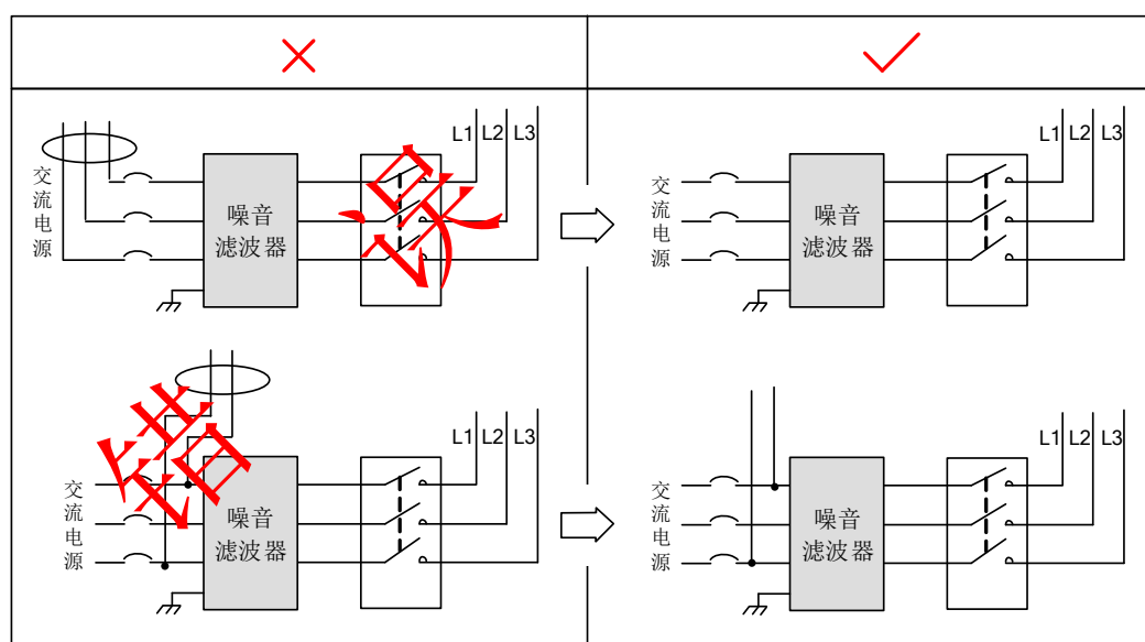
图4-13 噪音滤波器输入与输出配线分离走线示意图
