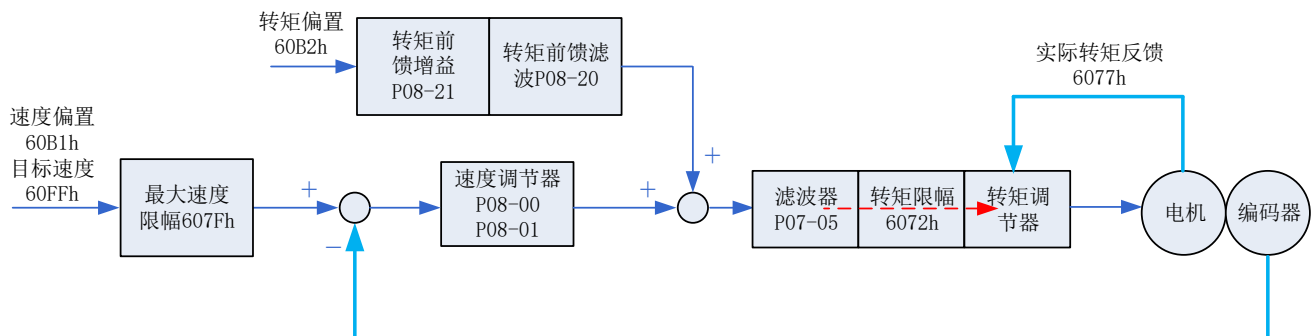
图 7-24 同步周期速度模式（csv）配置框图
