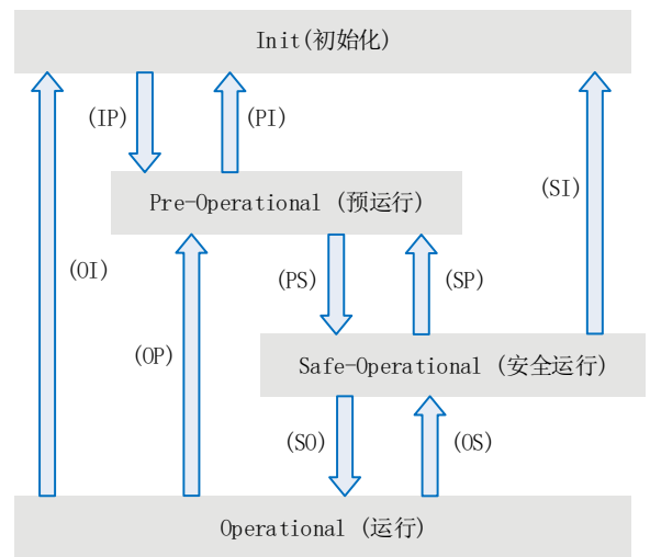
图 6-4 EtherCAT 状态机
