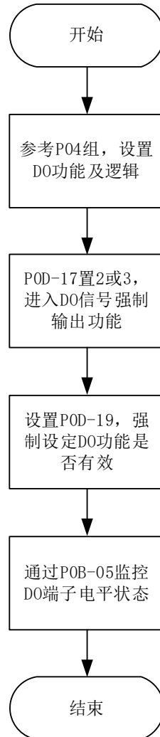
图 5-10 D0 信号强制输出设定步骤示意图
