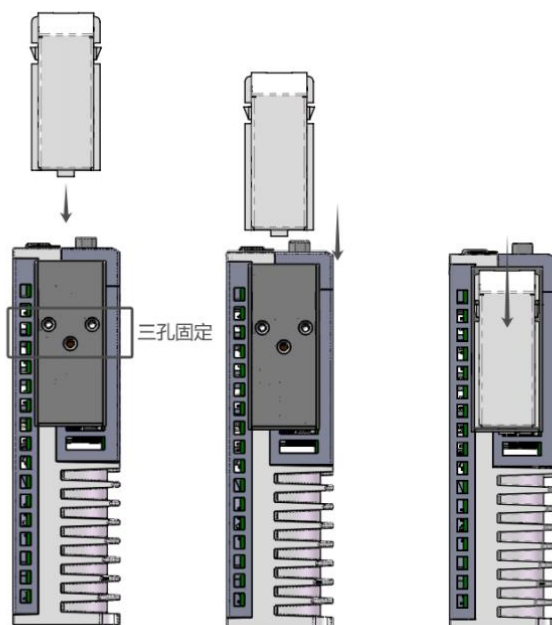
多圈编码器电池盒安装示例 2
