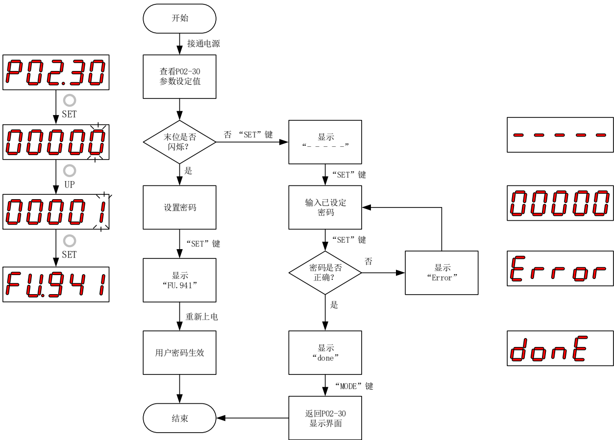
图 5-5 用户密码设定步骤示意图
