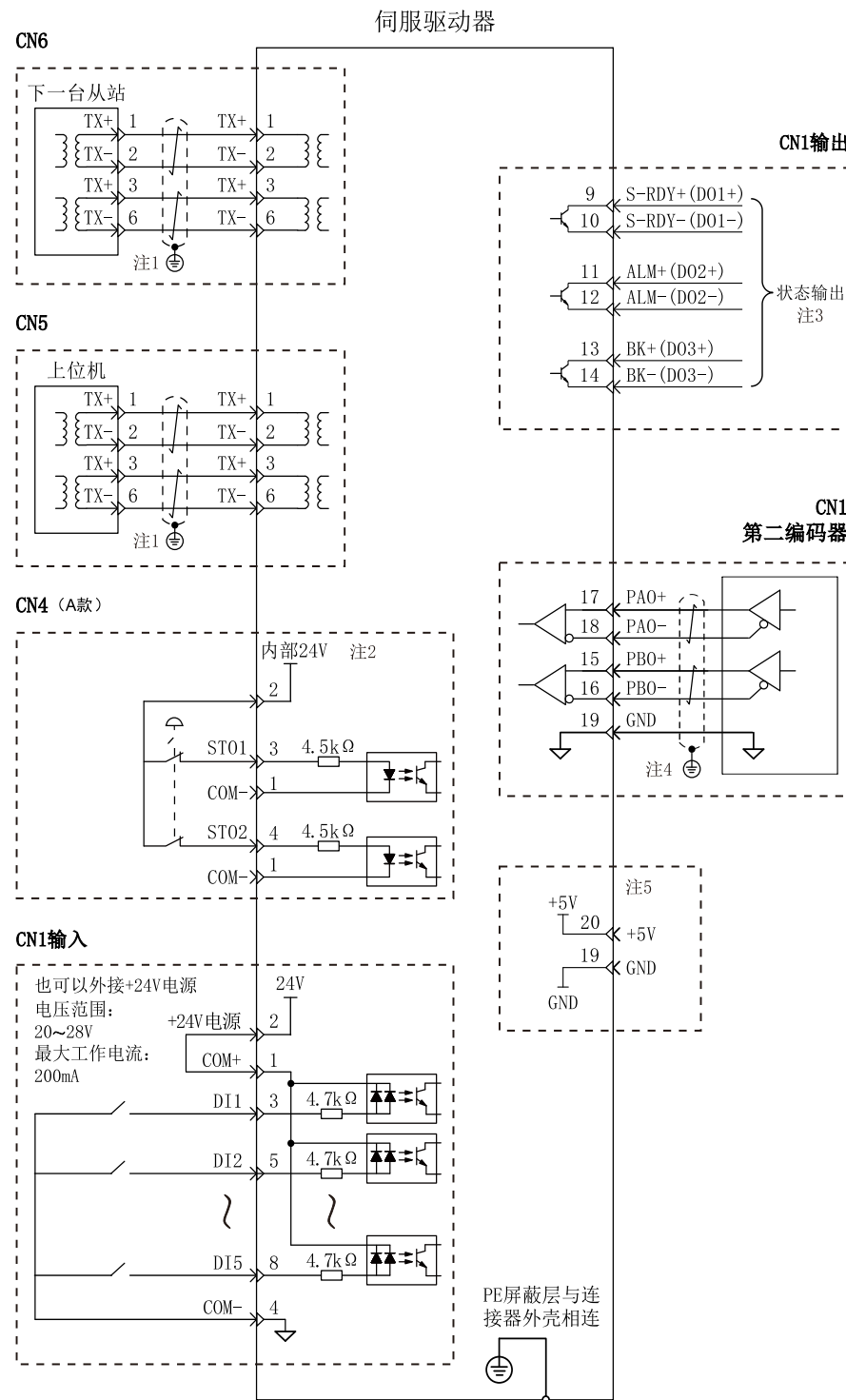
图 4-18 总线配线示意图
