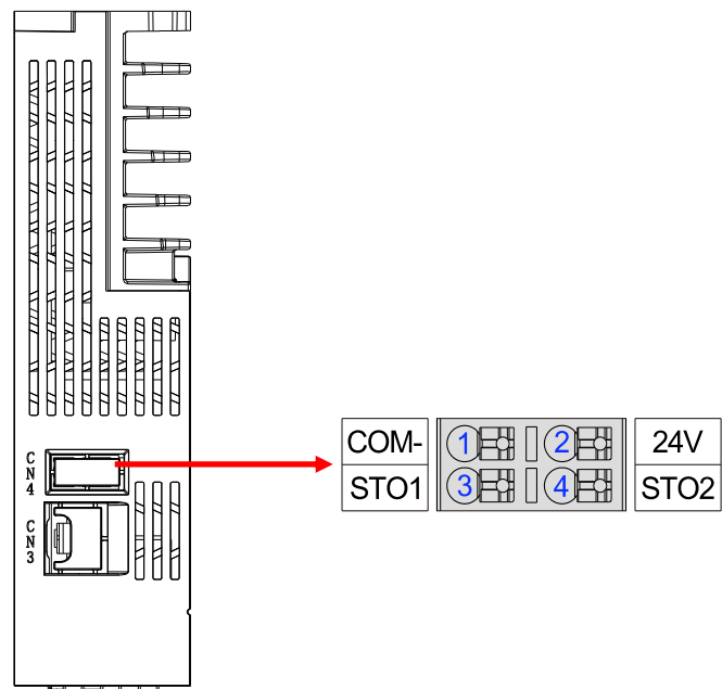
图4-10 推荐线缆示意图
