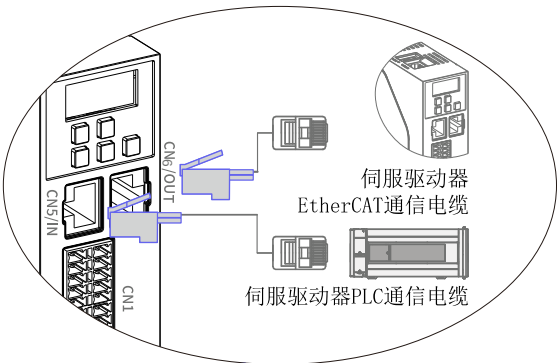
图4-11 通信配线示意图
