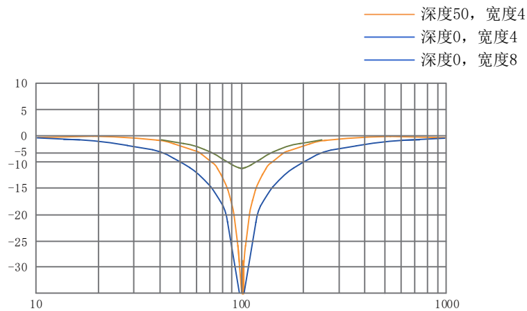
图 9-15 陷波器频率特性
