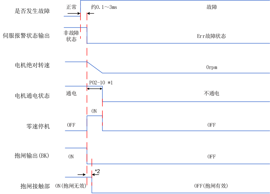
图7-16 故障2(带抱闸)时零速停机方式自由停机状态时序图
