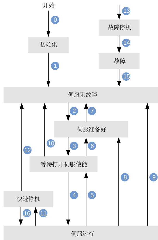
图 7-21 CiA402 状态机切换图
