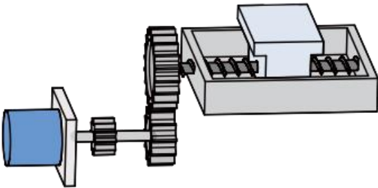
图 7-36 滚珠丝杠传动机构示意图
