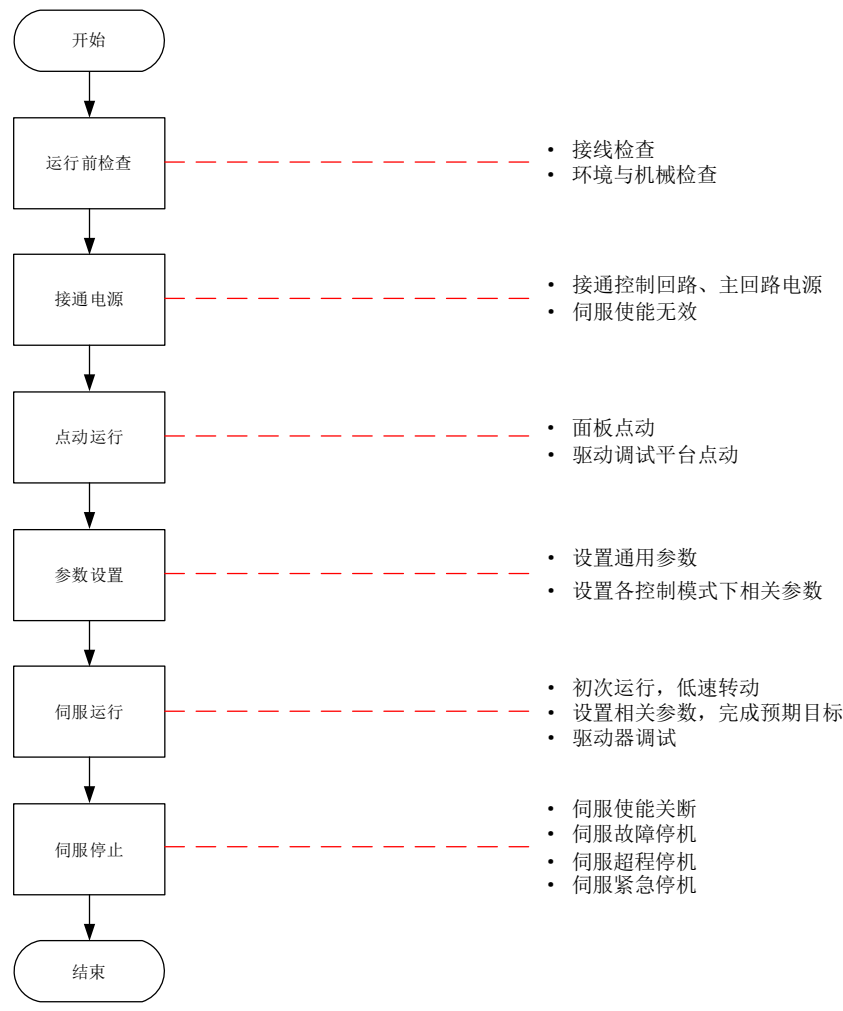
图 7-2 伺服设定流程
