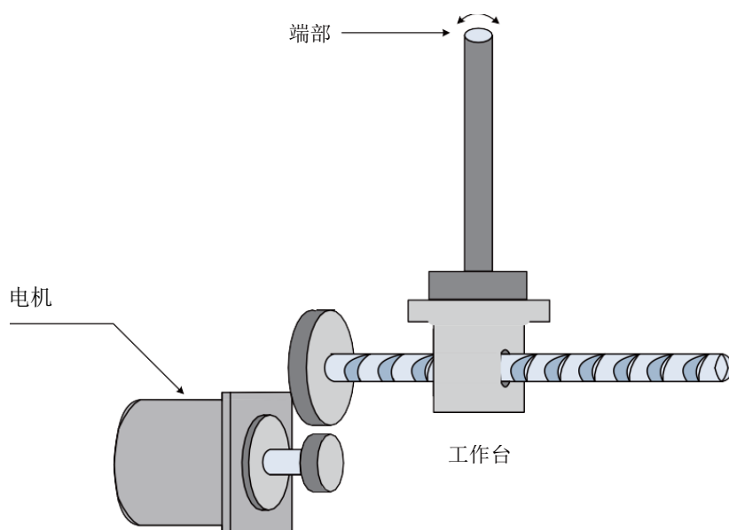
图 9-16 低频共振机械示意图
