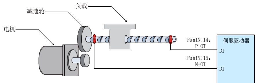
图 7-39 限位开关的安装示意图
