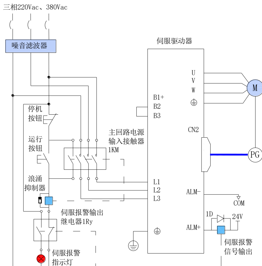
图4-5 三相220V、三相380V主电路配线
