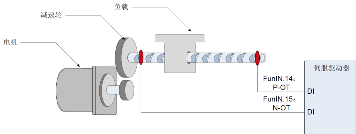
图7-20 限位开关的安装示意图
