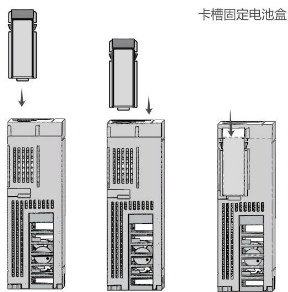
多圈编码器电池盒安装示例 1
