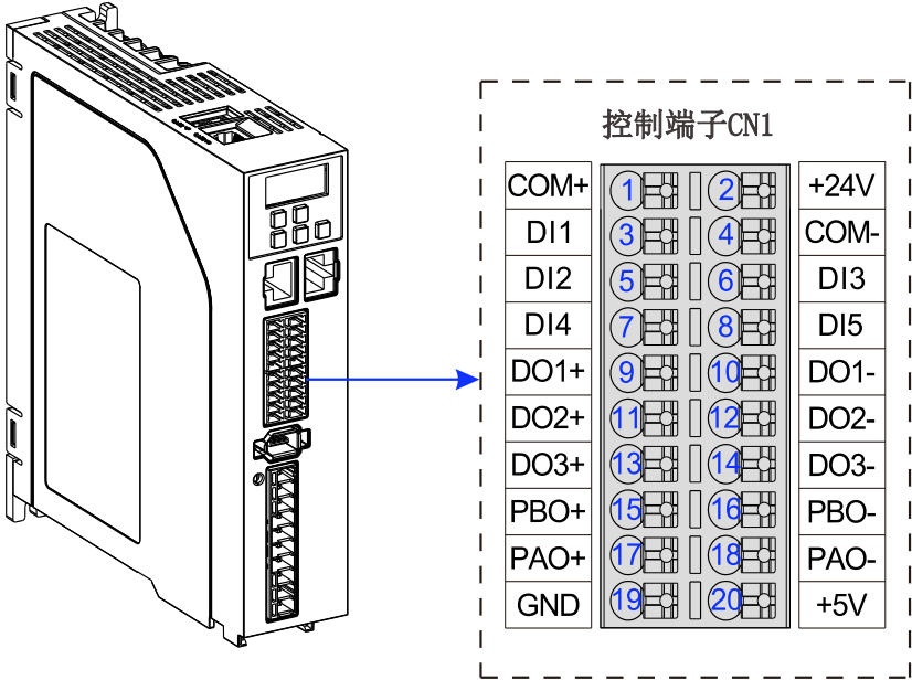
图4-8 驱动器控制回路端子连接器引脚分布图
