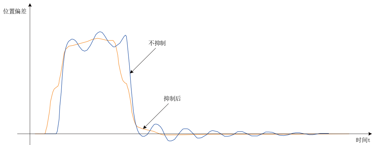
图 9-18 低频共振抑制效果图
