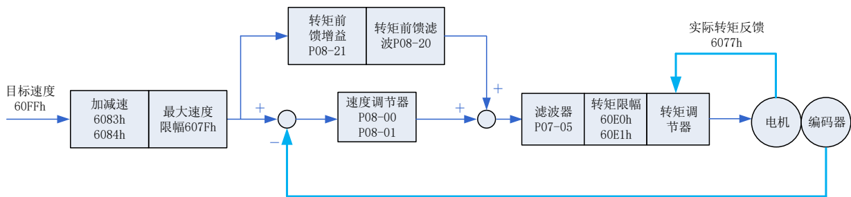
图 7-31 轮廓速度模式(pv)控制框图
