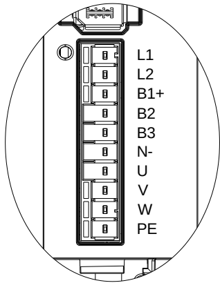
图4-2 伺服驱动器端子排布
