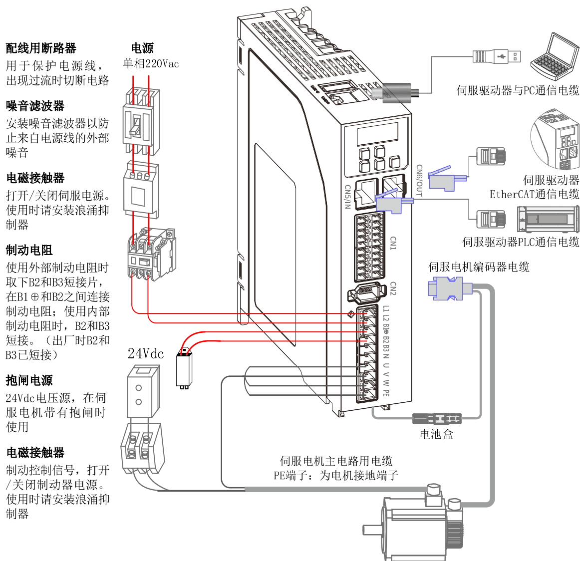
图 2-3 系统配线图举例
