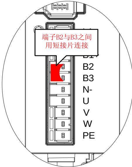
图7-10 内置制动电阻使用短接片示意图
