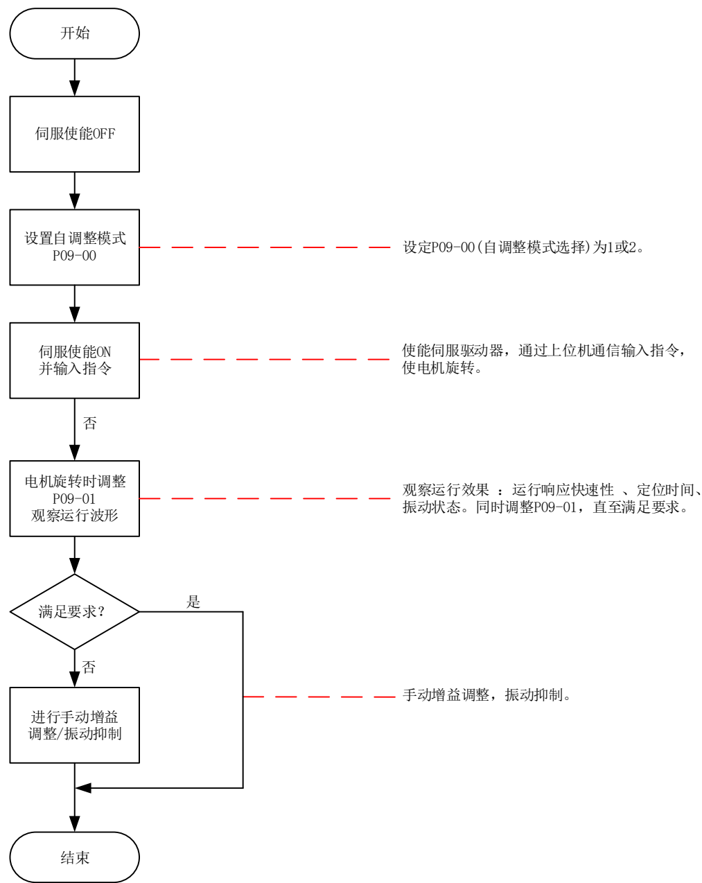
图 9-5 自动增益调整步骤
