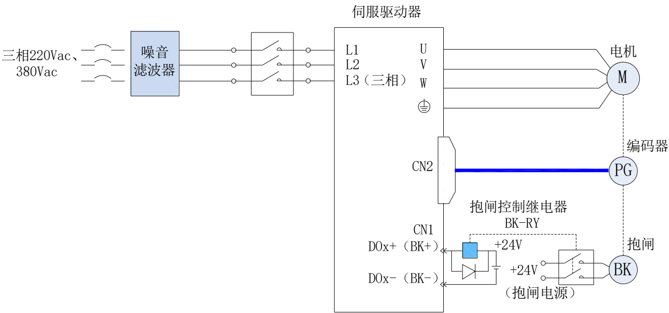
图 7-4 抱闸配线图
