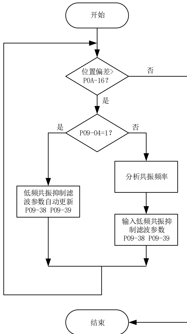
图 9-17 低频共振抑制滤波器使用步骤
