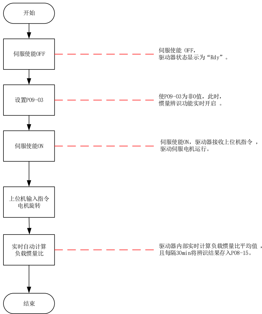
图 9-4 在线惯量辨识操作流程
