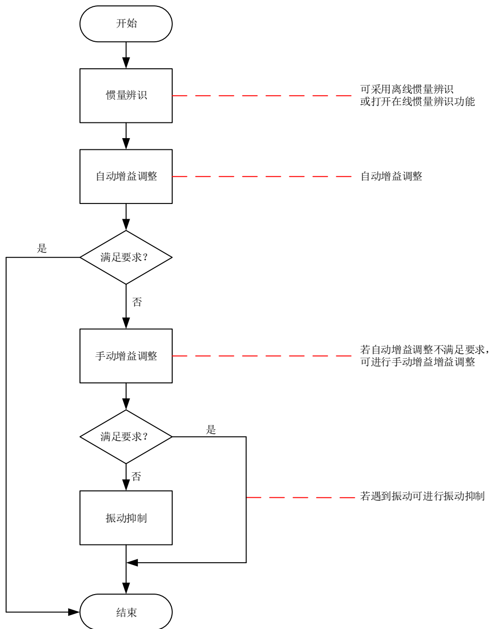
图 9-2 增益调整流程
