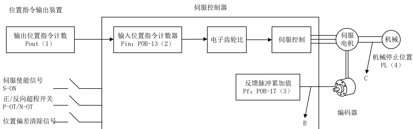
图 10-1 定位控制原理框图
