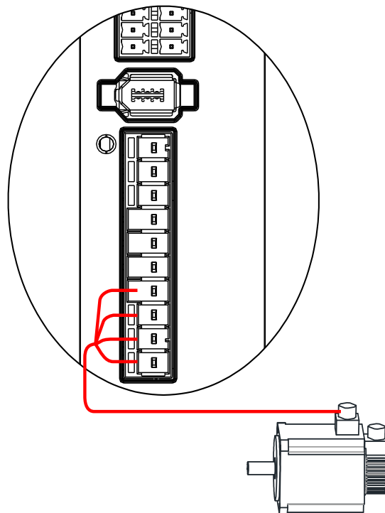
图4-6 伺服驱动器输出与伺服电机连接举例
