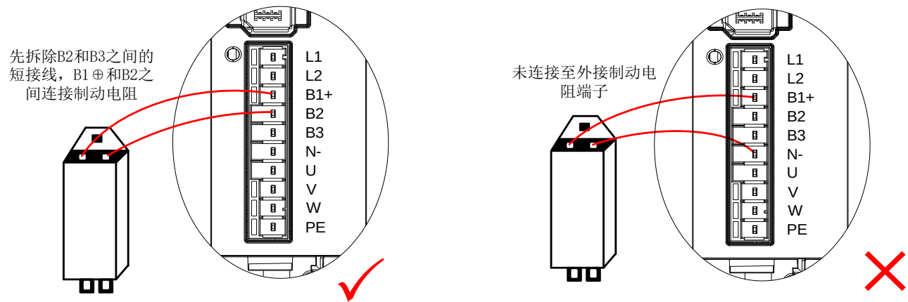
图7-9 外接制动电阻连接示意图
