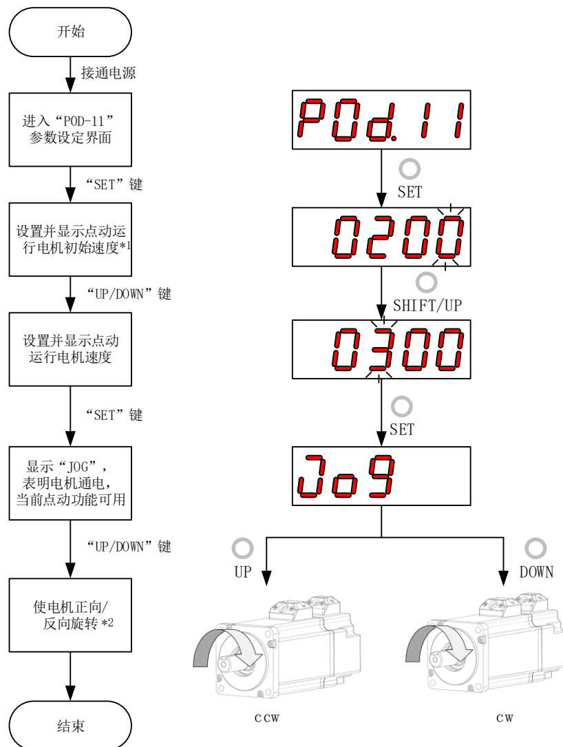
图 5-6 点动运行设定步骤示意图
