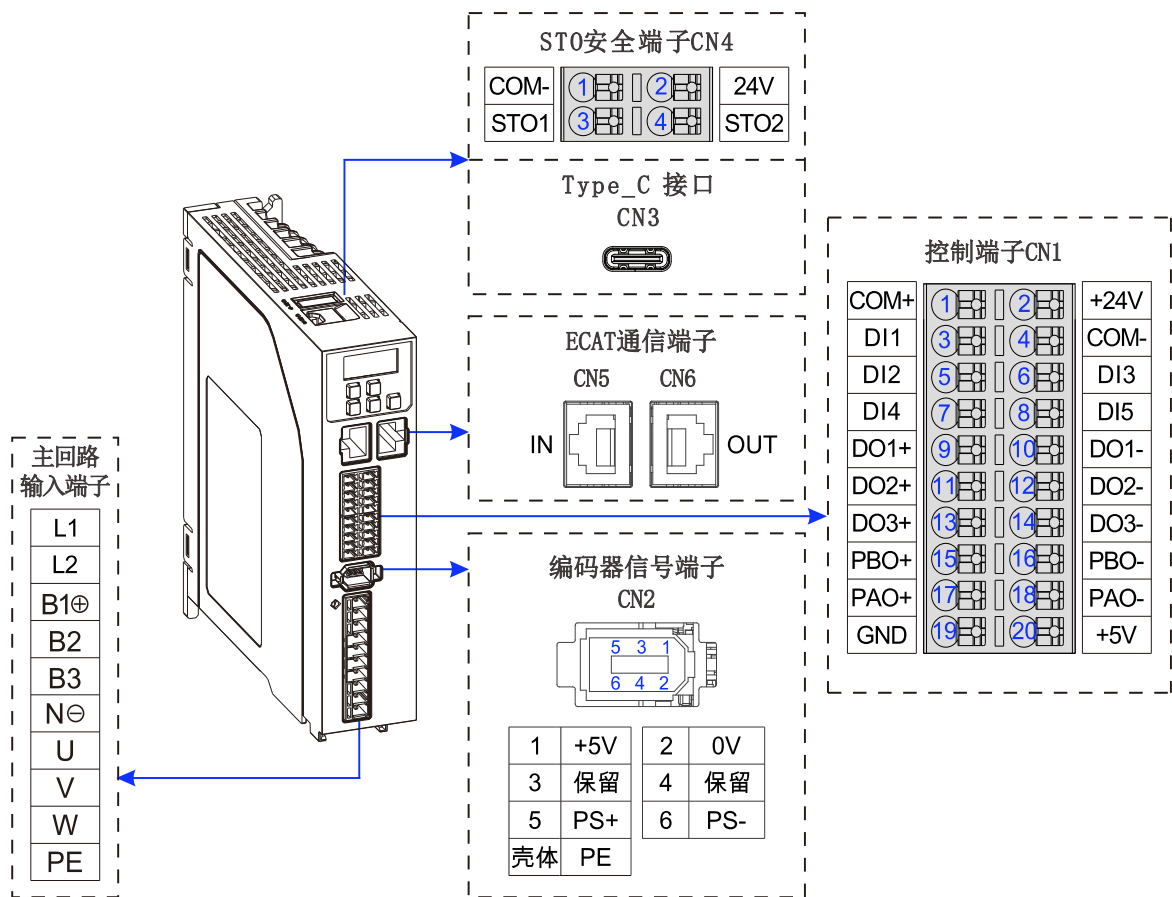
图4-1 伺服驱动器端子引脚分布图
