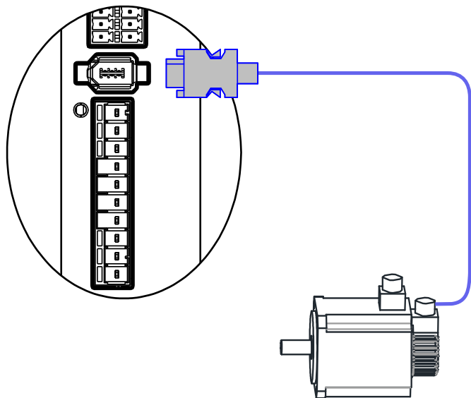
图4-7 编码器信号接线示例图
