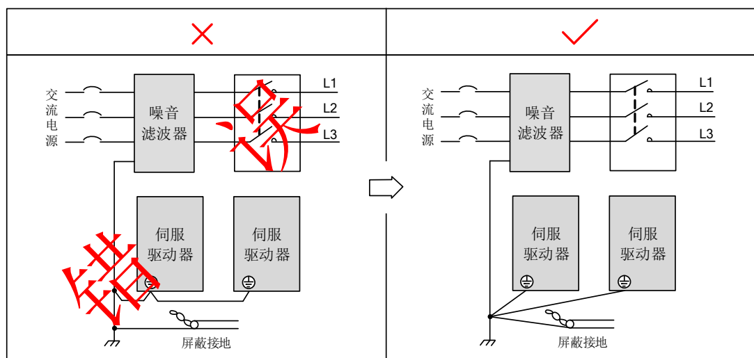
图 4-15 单点接地示意图
