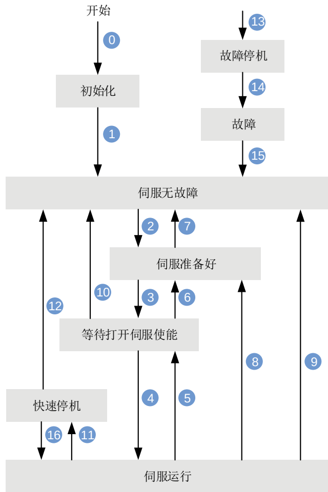
图6-6 CiA402状态机切换图
