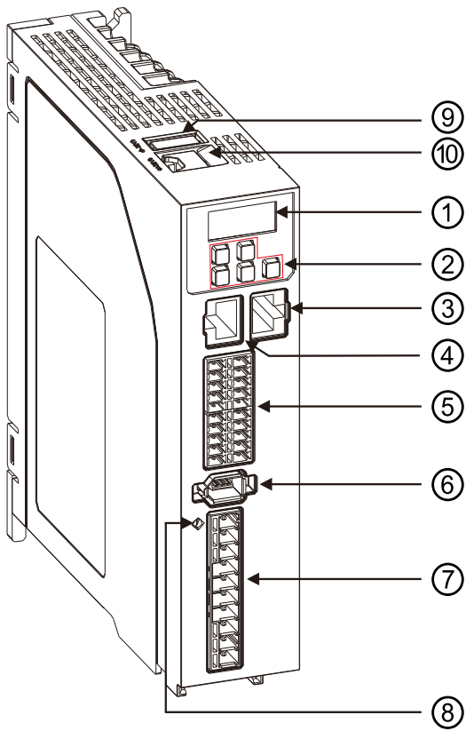
图 2-2 伺服驱动器组成
