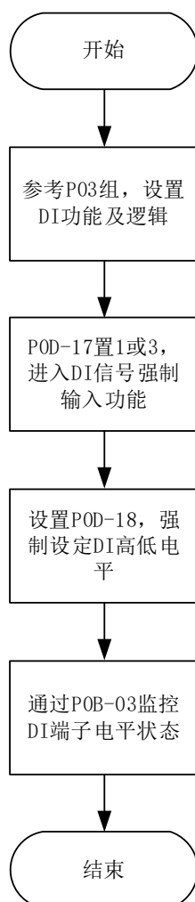
图 5-7 DI 信号强制输入设定步骤示意图
