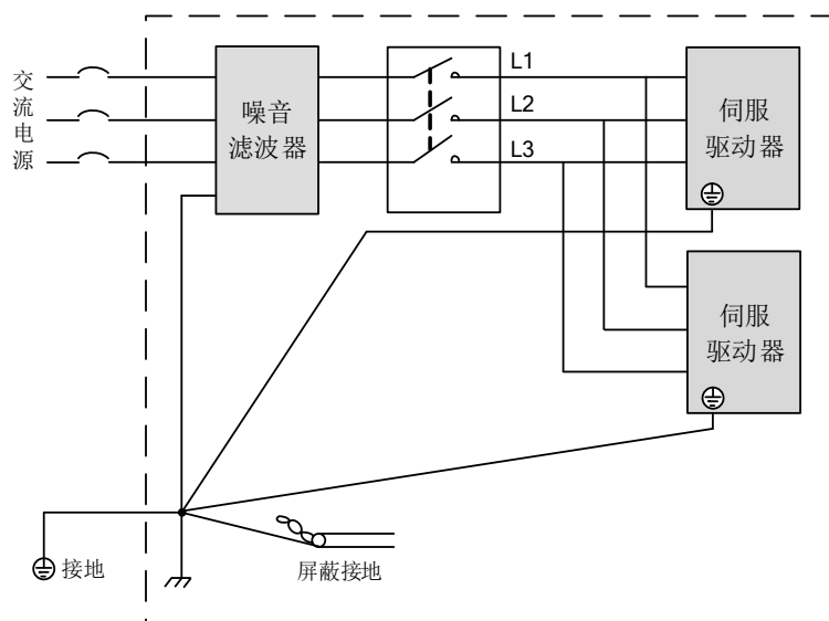
图 4-16 噪音滤波器地线处理示意图
