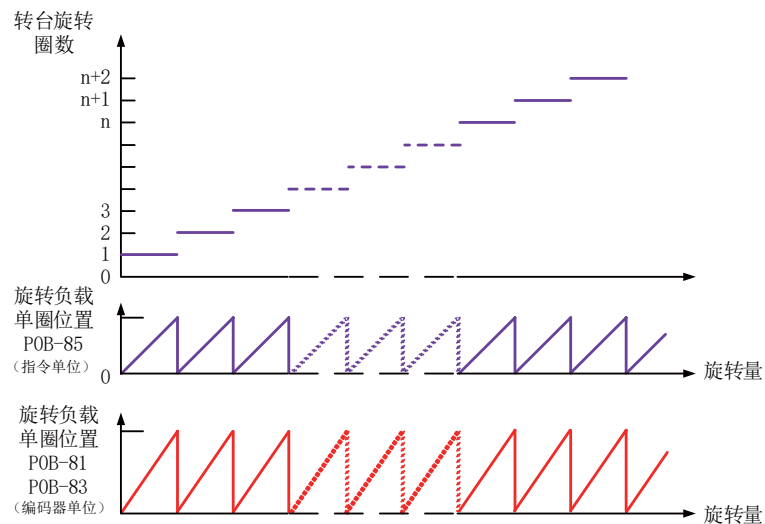
图 7-38 旋转负载单圈位置与转台位置对应关系示意图
