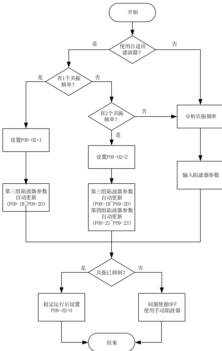
图 9-14 陷波器使用步骤
