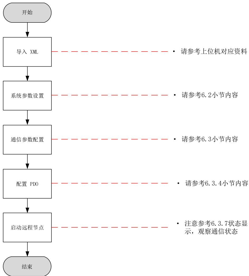
图 6-1 EtherCAT 使用设置流程图
