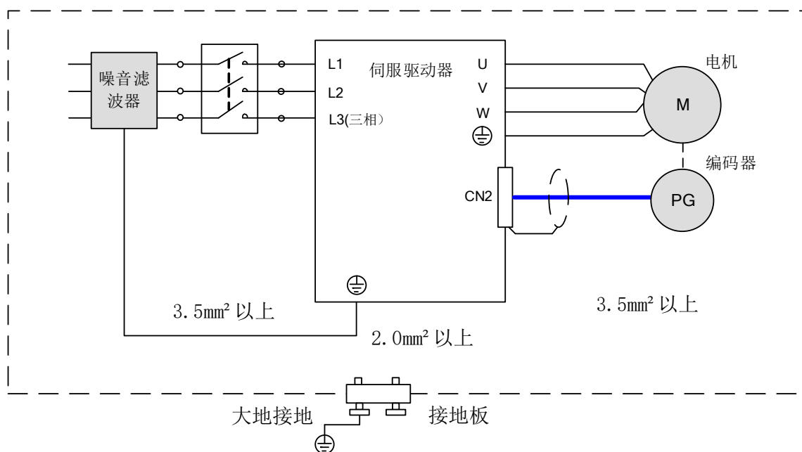
图4-12 抗干扰配线实例
