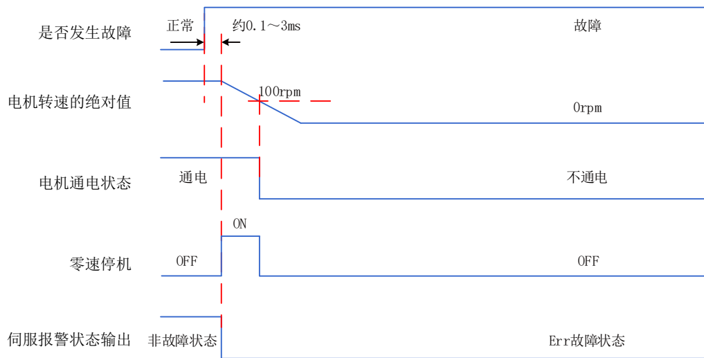
图7-15 故障2(非抱闸)时零速停机保持自由运行状态时序图
