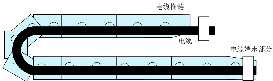
图 4-17 线缆保护链示意图
