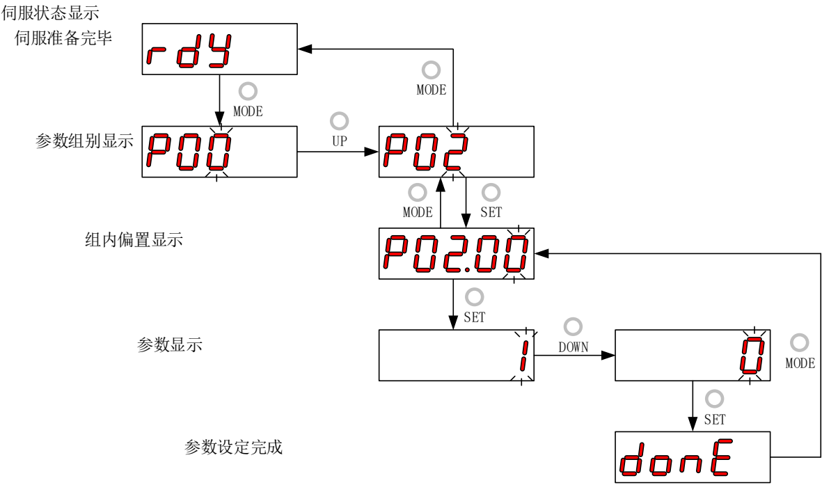
图 5-4 参数设定步骤示意图
