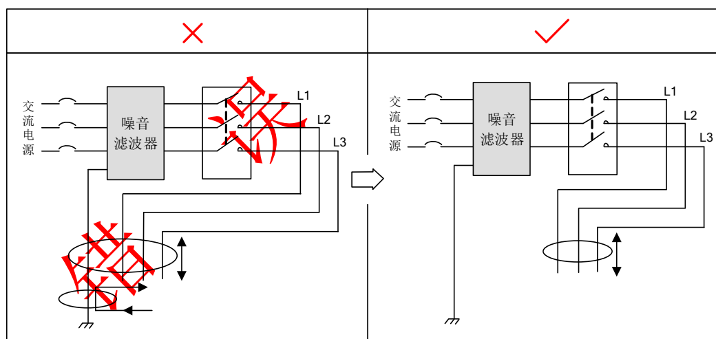
图4-14 噪音滤波器地线与输出配线分离走线示意图
