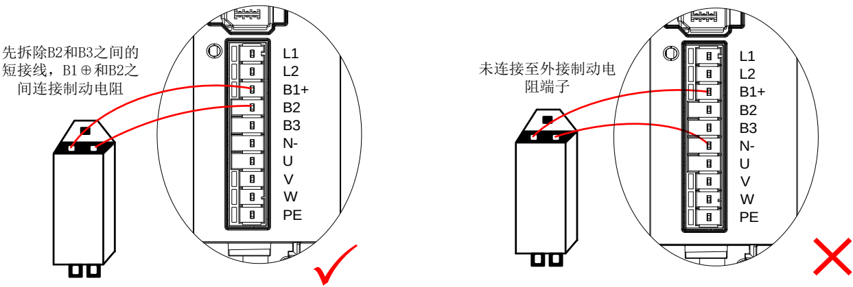
图4-3 外接制动电阻的连接示意图
