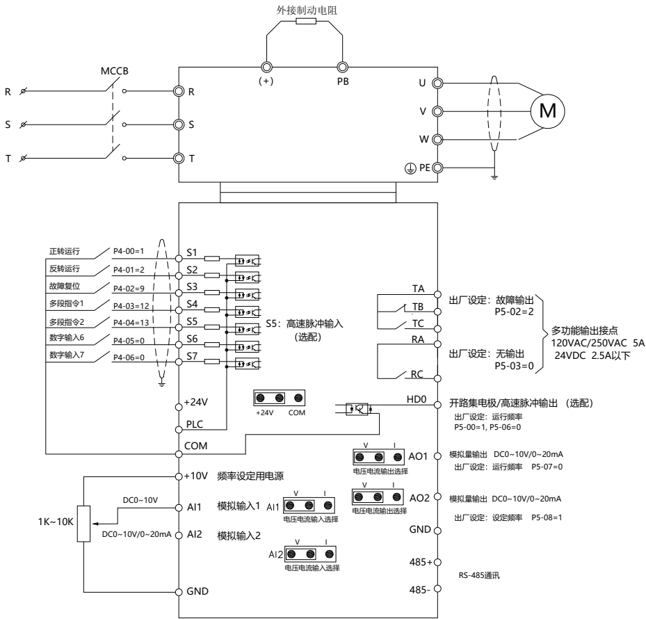
图 3-4 标准接线图
