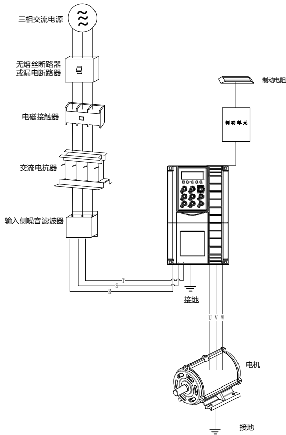
图 3-2 与外围器件连接示意图
